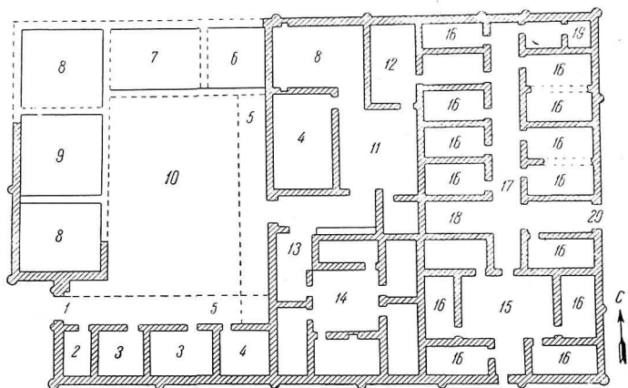
Рис. 17. План старого дома-усадьбы семьи Макеумлир, сохранившегося в поселке колхоза «Социализм» (Ханкинский р-н). Масштаб 1:100
