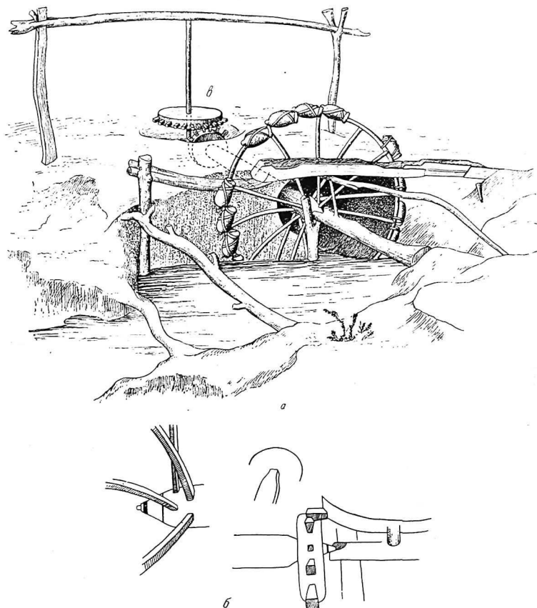
Рис. 3. Чигирь (схематический чертеж), Ханкинский р-н — общий вид; б — рисунки деталей; е — горизонтальное колесо, вращаемое рабочим снопом при помощи привода
