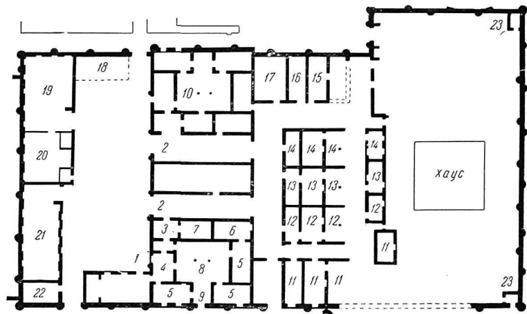
Рис. 18. План старого дома-усадьбы Матраим-бая, сына Саидмурата Бачмана, теперь правление колхоза им. Фрунзе (Хазараспекский р-н). Масштаб 1:100 (прежнее назначение помещений установлено при помощи местных жителей — стариков)
