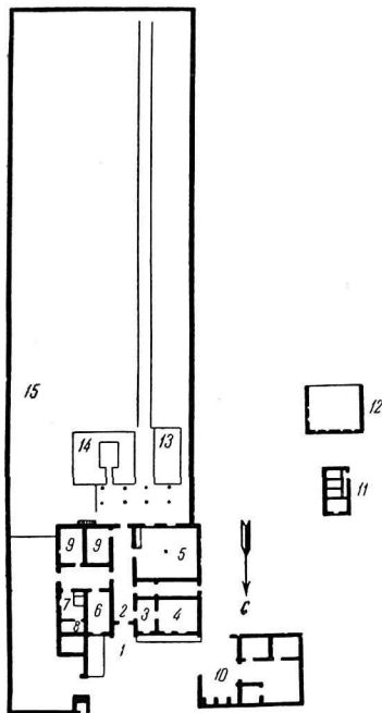
Рис. 32. План усадьбы Атабая Курбанова. Колхоз им. Сталина (Каш-Купырский р-н). Масштаб 1 : 200
