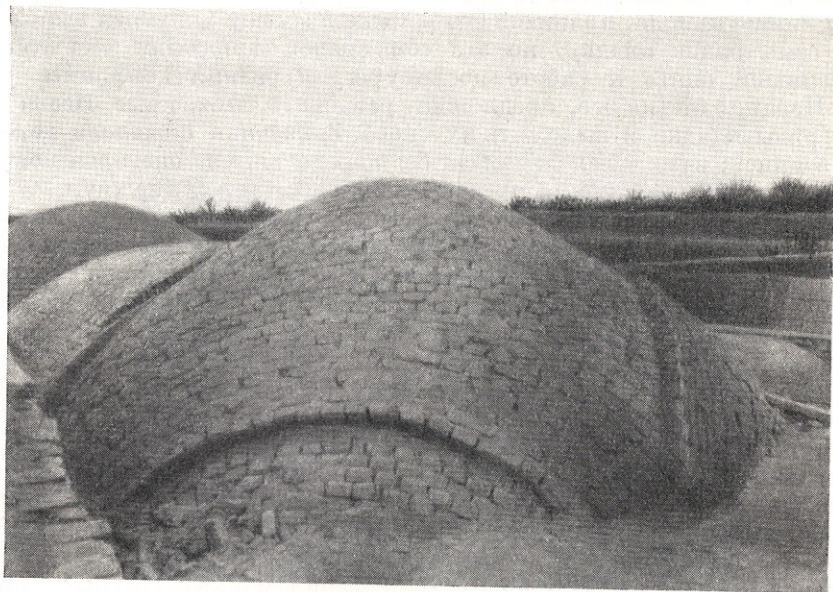
Рис. 29. Купол «балхи» с утолщенными полосами «зарба» в одном из помещений бани колхоза имени «Правды» под Андижаном
