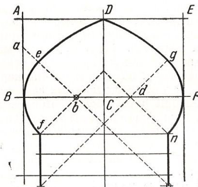
Рис. 42. Вычерчивание кривой купола «кафаса»
