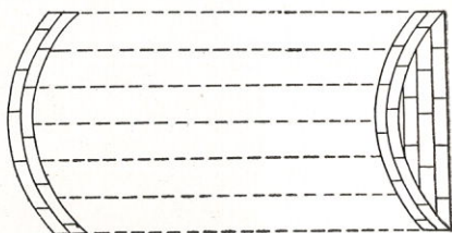
Рис. 31. Рисунок свода «зарбалик-гумбаз». По чертежу усто Юсуф Али Мусаева
