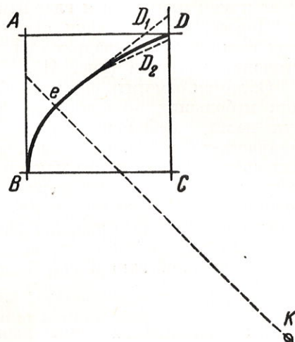
Рис. 40. Способ вычерчивания арок повышенного и пониженного подъема
