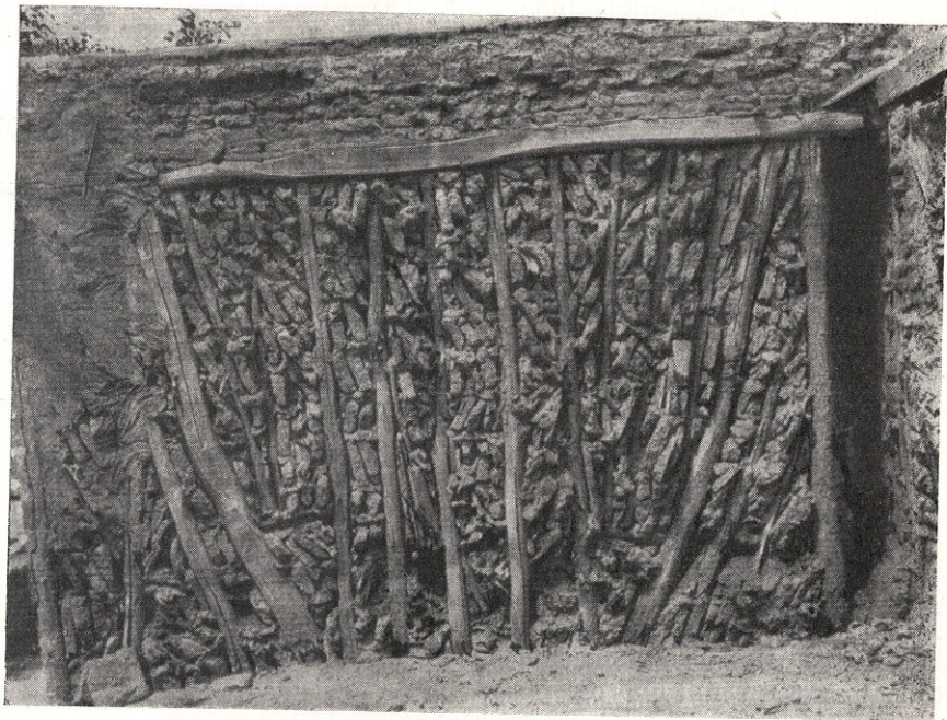
Рис. 17. Каркасная стена с подкосами и распорками в самаркандском жилом доме третьей четверти XIX в. (негатив в Музее искусств УзССР)
