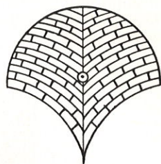
Рис. 34. Схема паруса «кафтар думи гаджик». По чертежу усто Юсуф Али Мусаева
