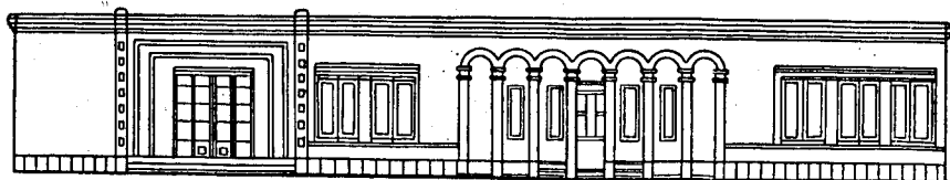
Главный фасад
