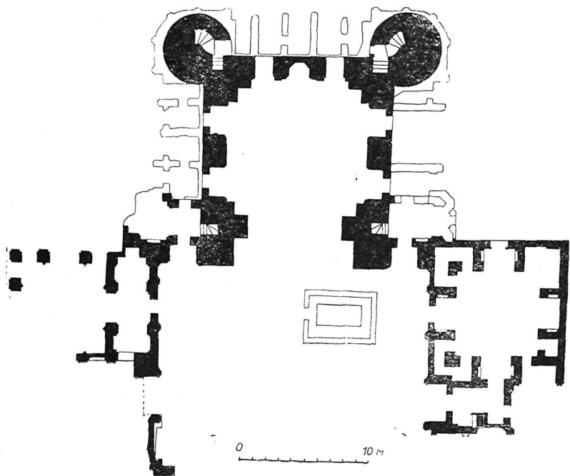
34. План мечети (состояние на 1947 г.)
