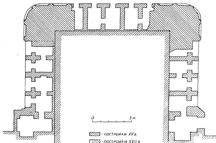
35. План цокольного этажа (реконструкция).
