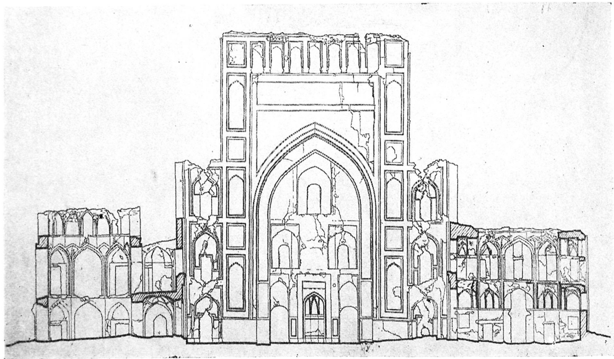
38. Фасад дворового айвана и разрез через дарсхану
