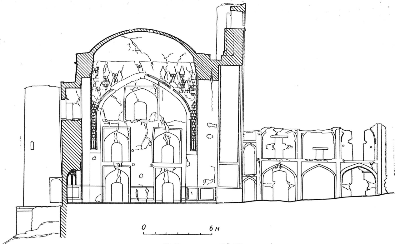
39. Разрез по главной оси.
