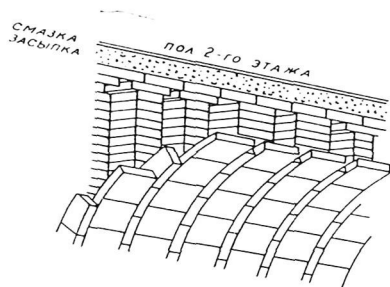
26. Свод в северо-западной дарсхане.
