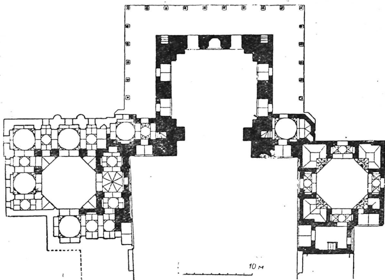
36. План I этажа (реконструкция).
