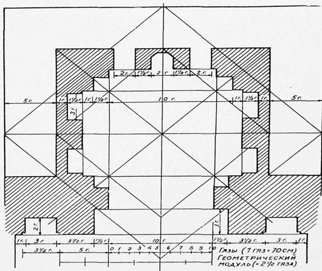
41. Анализ пропорций плана главного здания мечети.
