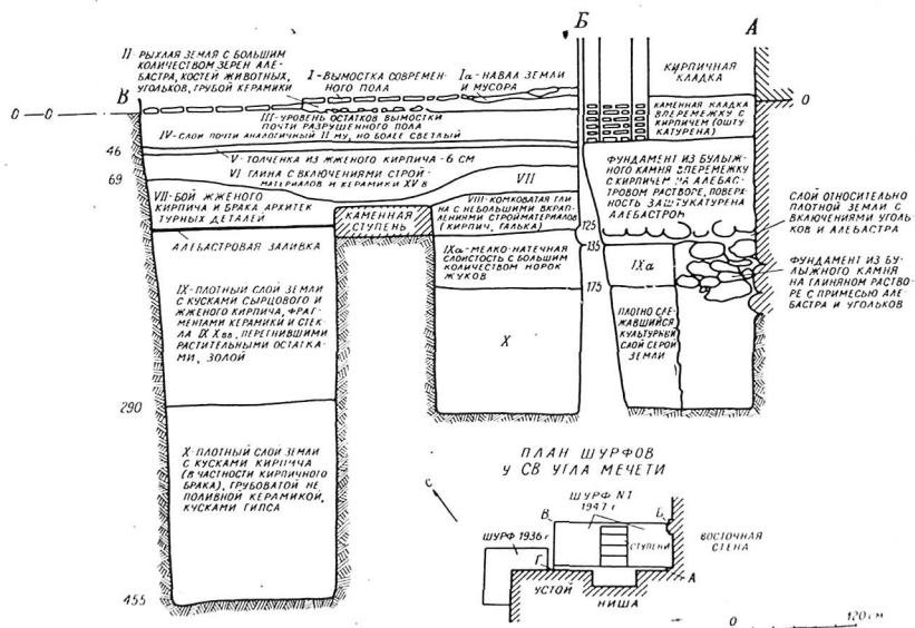
18. Фундаменты, вскрытые у северо-восточного угла двора мечети (шурф № 1).
