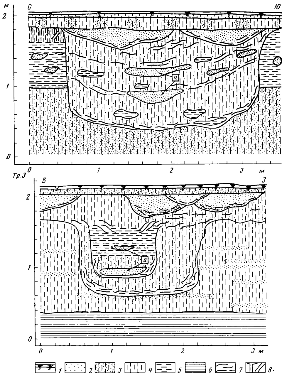
Рис. 4. Поперечные разрезы через оросители 1-го и 2-го порядка у Мадау-депе 1 — современный почвенный горизонт; 2 — песок; 3 — супесь; 4 — суглинок; 5 — легкая глина; 6 — глина; 7 — глинистые прослои; 8 — ходы насекомых
