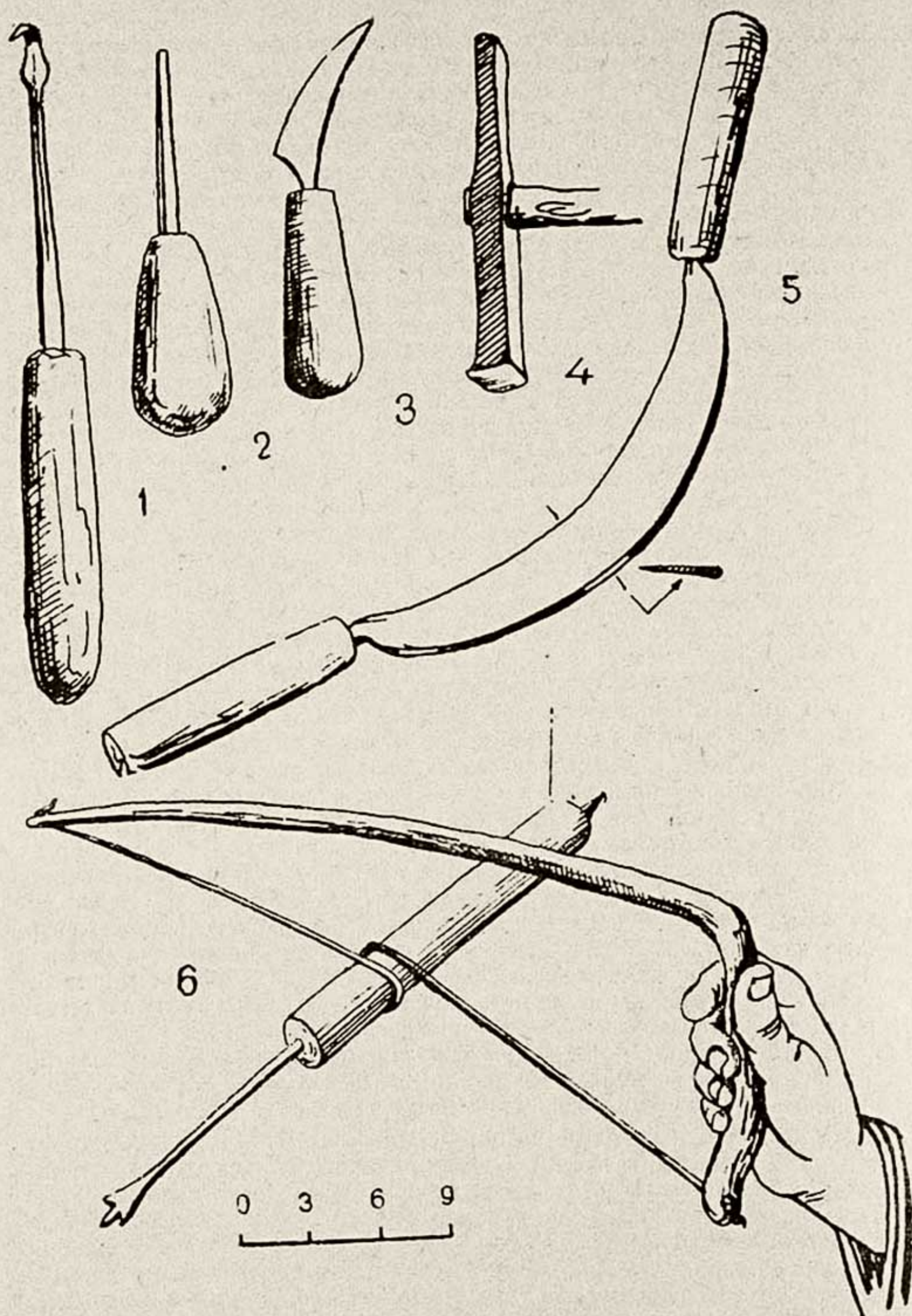
Рис. 57. Орудия труда ремесленников из Дарваза: 1—қошуққан—нож с загнутым лезвием для выделывания ложек, к. Пшихаря (КП 156—184); 2—парма—плоское шило, оттуда же (КП 156—183); 3—чари-бур—сапожный нож, к. Егид (КП 273—362); 4—ховискча—небольшой молоток, оттуда же (КП 273—235); 5—досранд—скобель для обстрагивания поверхности балок и т. п., к. Пшихаря (КП 156—210); 6—обпарма—сверло, вращаемое лучком—камончик, к. Егид (КП 273—189).
