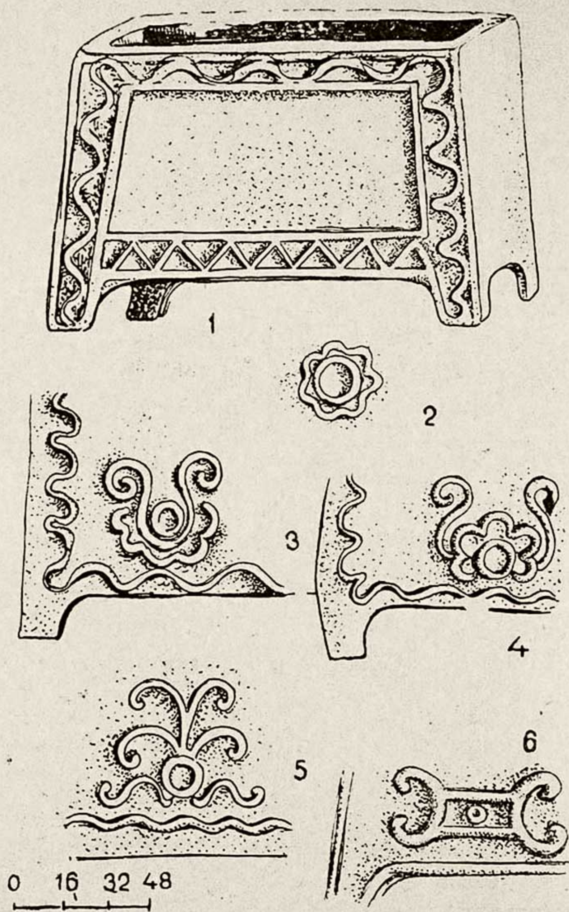
Рис. 55. Глиняные лари:
