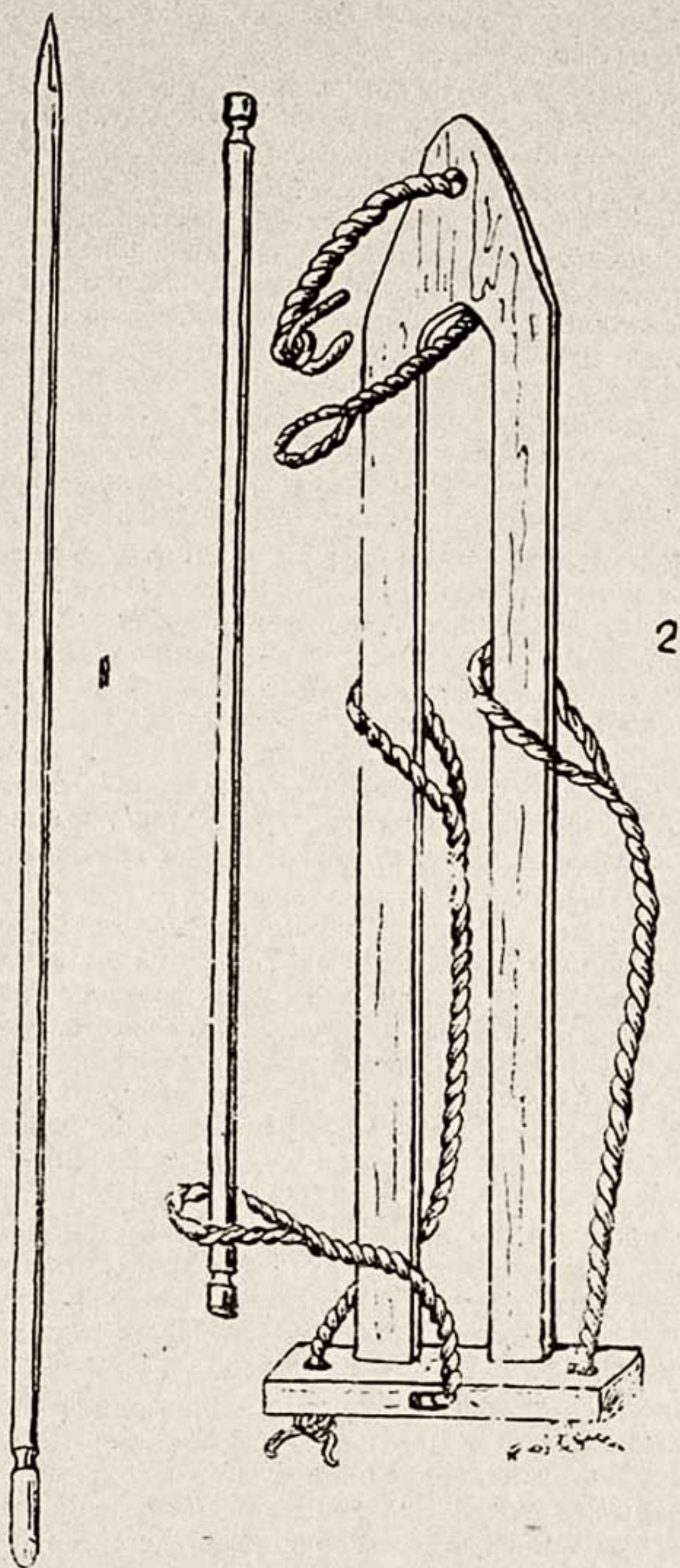
Рис. 21. Деревянные приспособления для переноски на спине снопов хлеба и трав: 1—сик, Дарваз, к. Егид; 2—кош, Дарваз, к. Пшихарв.
