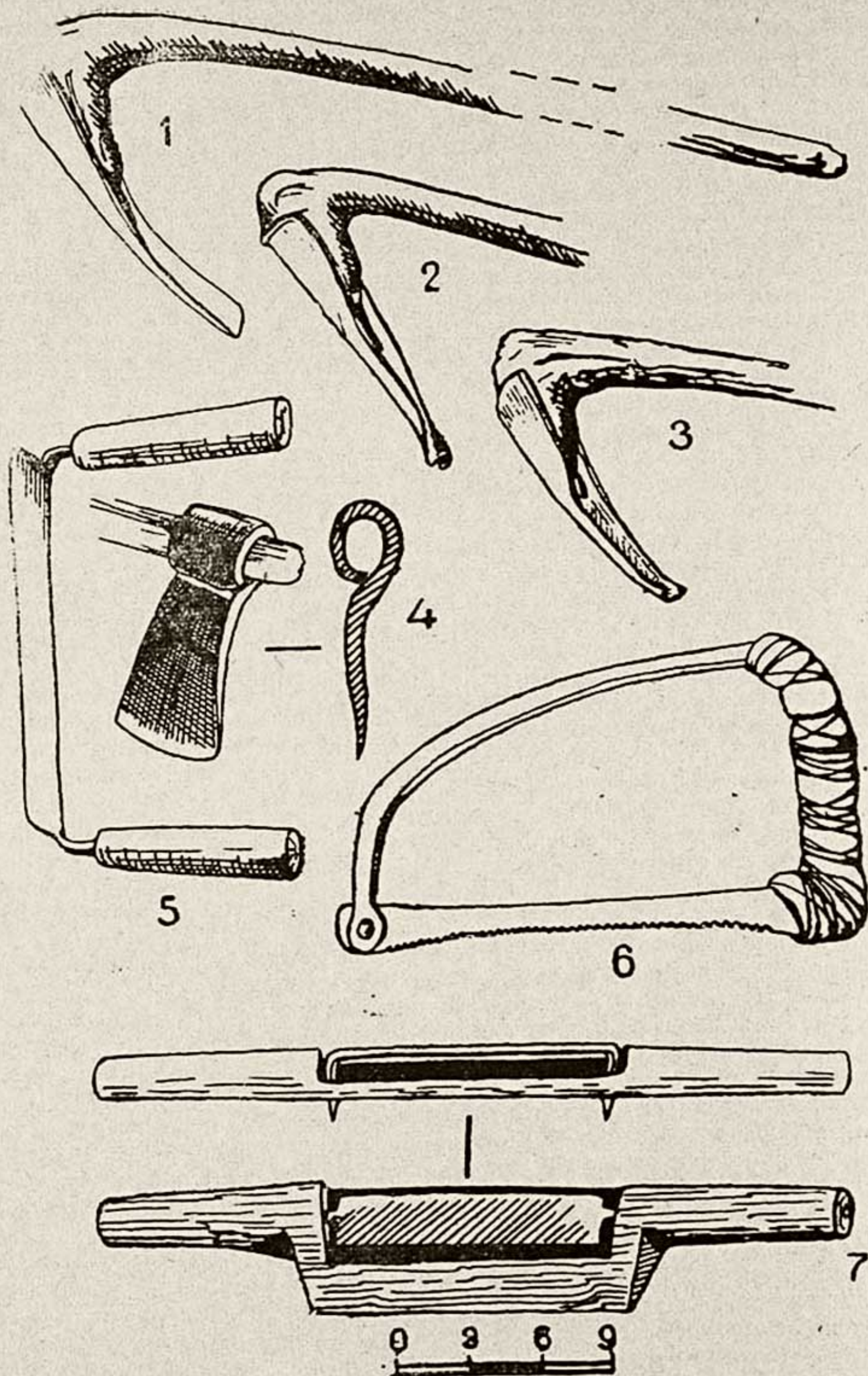
Рис. 56. Орудия труда деревообделочников из Дарваза: 1— теша —тесло, к. Пшихарв (КП 156—122); 2— тешаи чапновак —тесло с лезвием желобком наружу, отсюда же (КП 156—164); 3— тешаи новак —тесло желобком для вытачивания внутренности деревянных башмаков, к. Егид (КП 273—123); 4— таварча —топор, отсюда же (КП 273—151); 5— леса —скобель для обстрагивания балок, отсюда же (КП 273—165); 6— арраи шона —пилка для выделки гребней, к. Егид (КП 273—219); 7— ранда —рубанок, отсюда же (КП 273—147).
