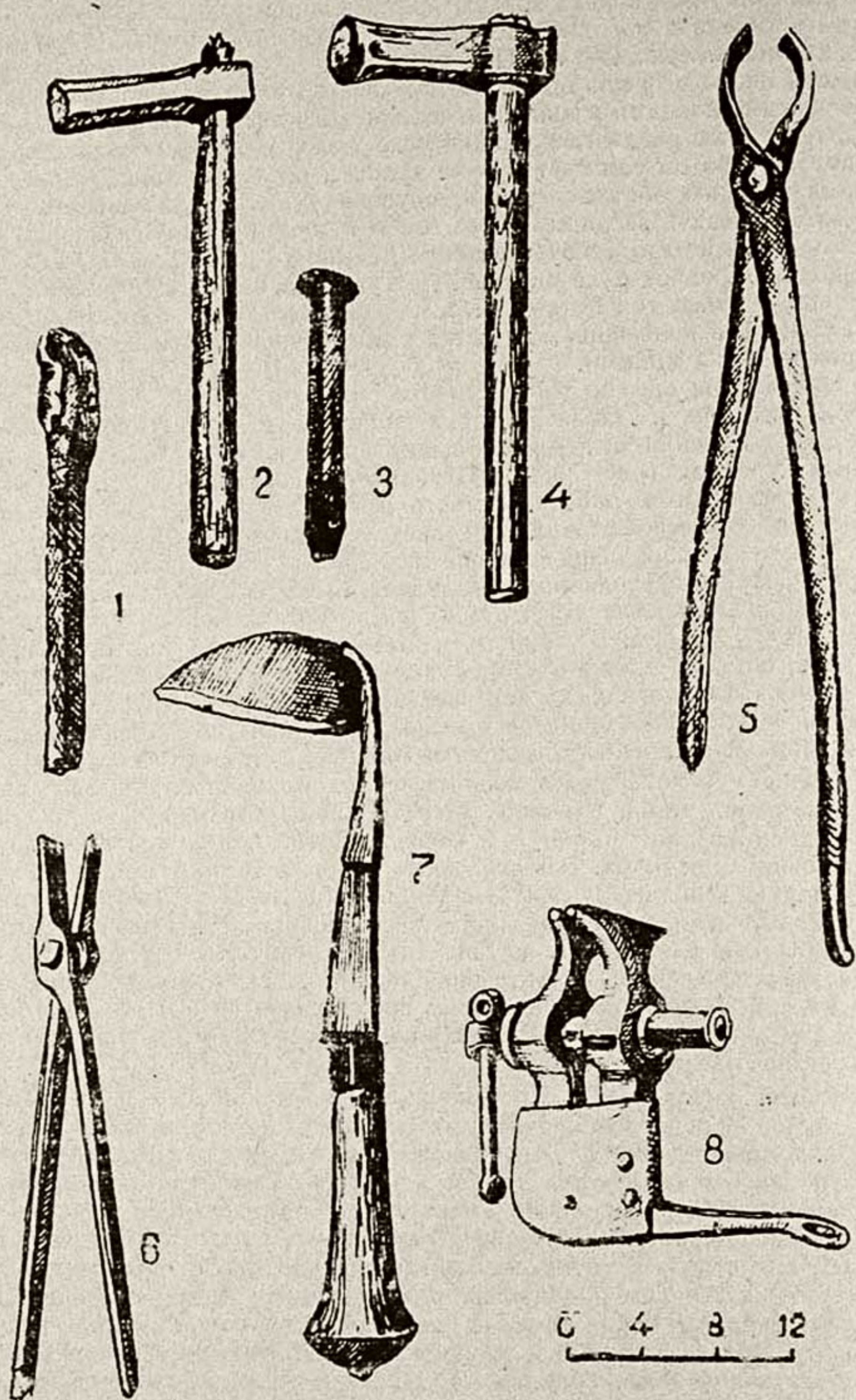
Рис. 39. Кузнечные инструменты из Каратегина, к. Шуль: 1—мехқолаб—металлический стержень с отверстием дляковки гвоздей (КП 210—3); 2—болиқа—молоток (КП 210—10); 3—қаламак—зубило (КП 210—6); 4—хоиск—молот (КП 210—9); 5—качанбур—клещи с загнутыми концами (КП 210—5); 6—анбур—клещи-плоскогубцы (КП 210—4); 7—сумғарош—нож-скребок для зачистки копыт при подковывании (КП 210—7); 8—гиро—тиски местной кустарной работы (КП 210—2).
