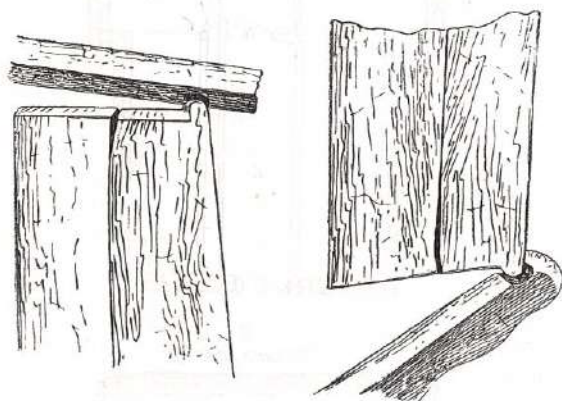
Рис. 27. Детали скрепления двери с притолокой и порогом.
