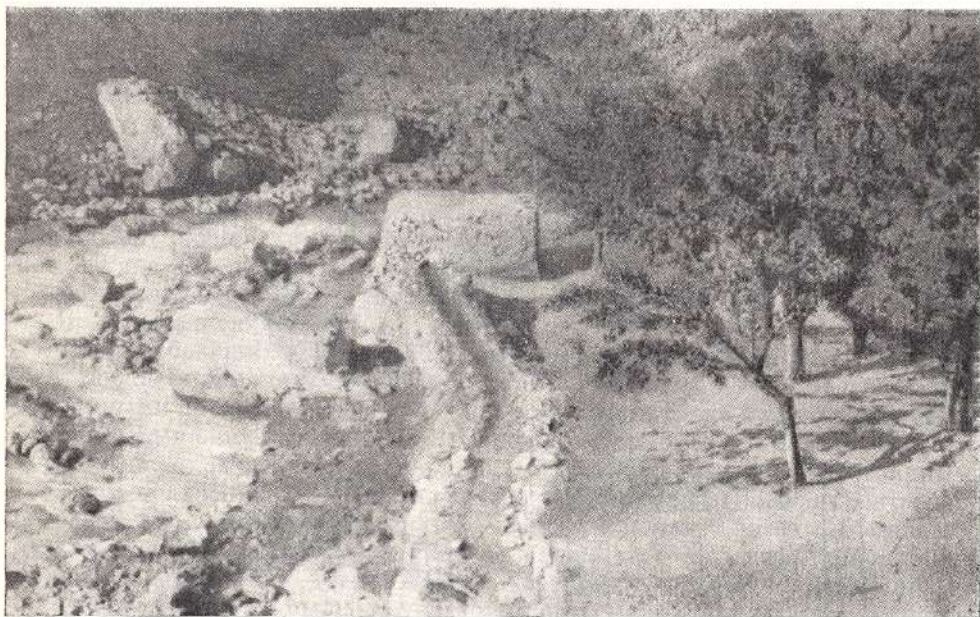
Рис. 10. Водяная мельница «хаёрг».
