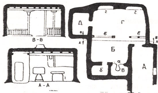
Рис. 42. План и разрез дома Азимова Махсума, к. Дарг:
