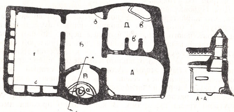
Рис. 35. План и разрез дома Абуева Азима, к. Вору: А — айвон; Б — прихожая — кавшарто ; В — очажное отделение — мур ( алавхона ); Г — чистое отделение — руи боло ; Д — кладовая — амбор ; а — очаг; б — яма-поглотитель — обрез ; в — ларь — хамба ; г — ниши в стене — ток .
