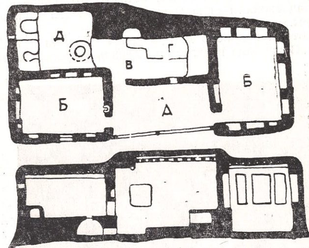
Рис. 33. План и разрез дома братьев Муллаевых, к. Кули-Дахана, построен в 1960 г.: А — веранда — долун ; Б — помещение нового вида — хучра ; В — прихожая — куча ; Г — канна, используется как место для стряпни; Д — очажное отделение — мур .
