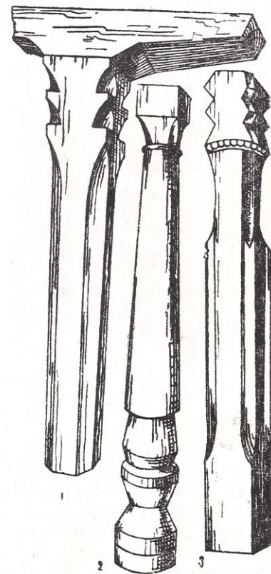
Рис. 68. Колонны жилища: 1 — к. Искодар; 2 — к. Ревомутк; 3 — к. Дарх.
