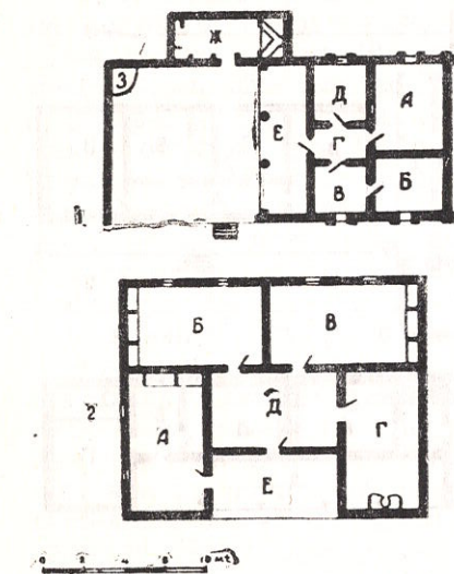
Рис. 52. Планы домов:
