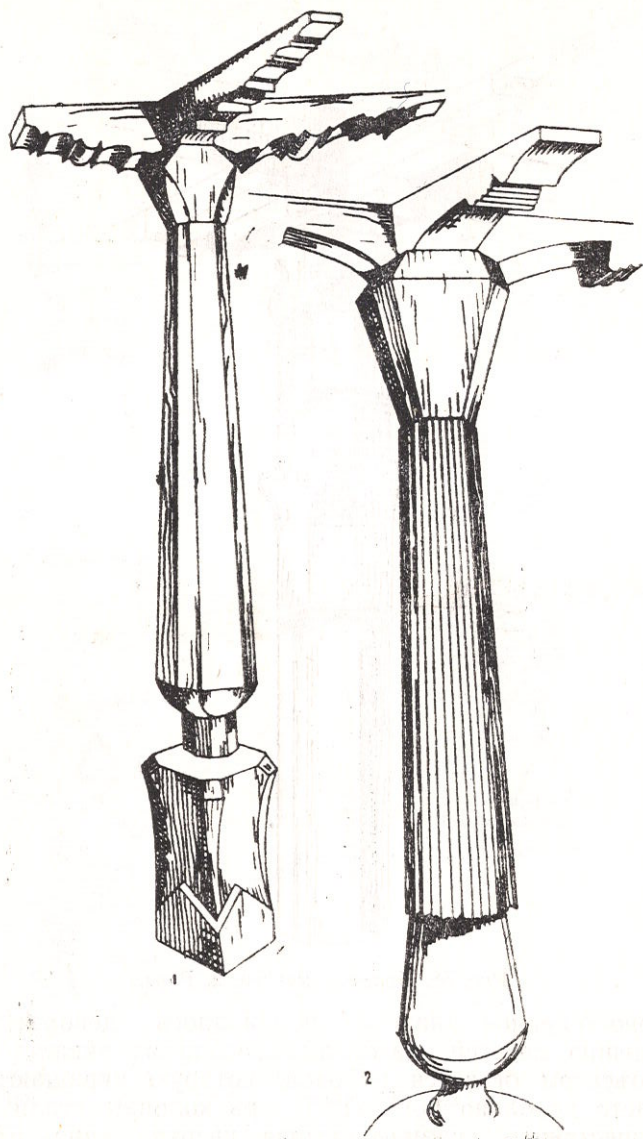
Рис. 59. Колонны мечети: 1 — к. Ревомутк; 2 — к. Дарх.
