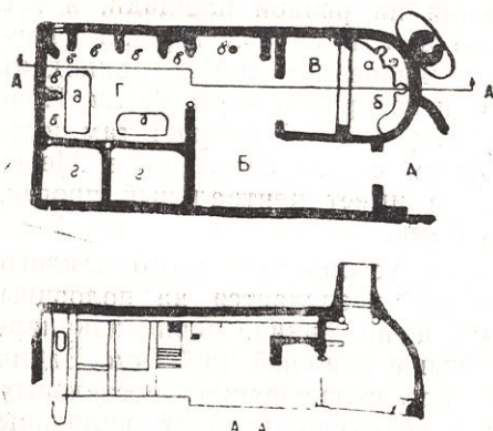
Рис. 44. План и разрез дома Бабаева Мурода, к. Газа:
