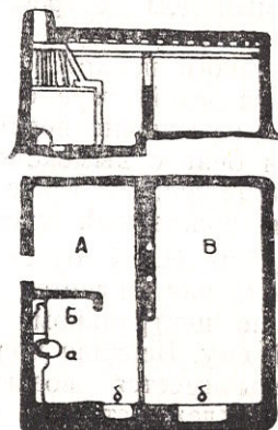
Рис. 45. План и разрез дома Хасановой Муслимы, к. Вору:
