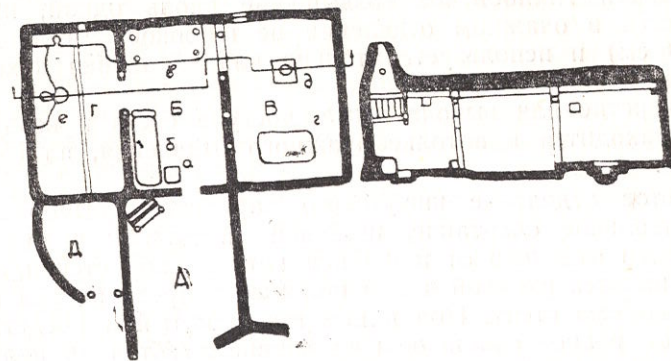
Рис. 36. План и разрез дома Кенджаевой Бибилатиф, к. Газза: А — айвон; Б — прихожая — кавшарто ; В — чистое отделение — руи боло ; Г — очажное отделение — мур ( алавхона ); Д — помещение для топлива — хезумхона ; а — яма-поглотитель — обрез ; б — возвышение для дров — суфай хезумгир ; в — скамейка для складывания постельных принадлежностей; г — яма-зернохранилище — чоу ; д — сандаль ; е — очаг.
