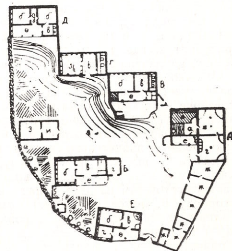
Рис. 24. План дома Каримова, состоящего из нескольких жилых комплексов и мехмонхон, построенных в разное время, к. Фароб:
