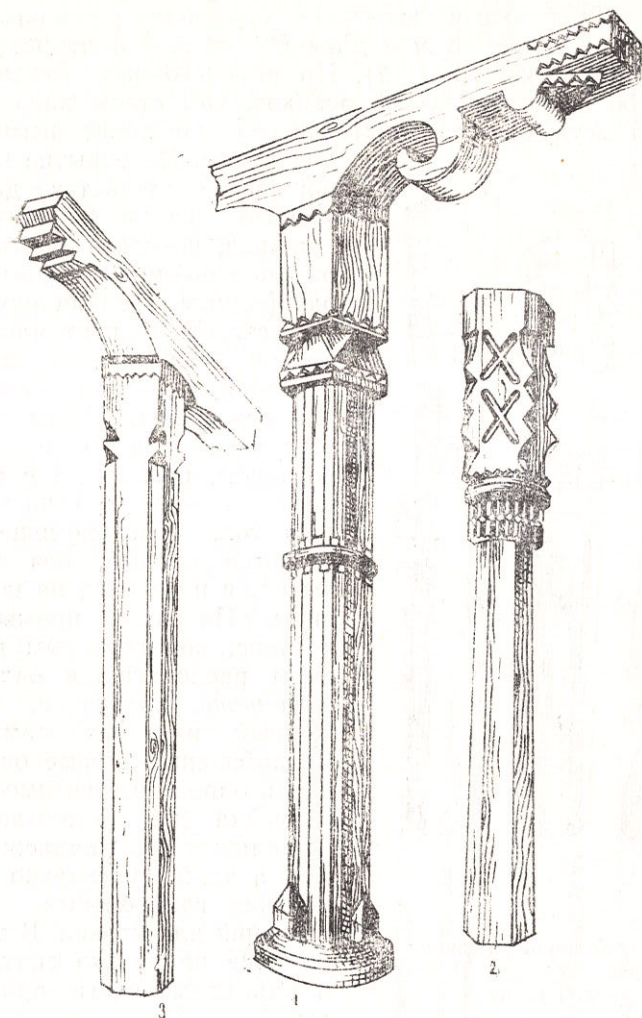
Рис. 66. Колонны жилища: 1 — к. Курут; 2 — к. Худгиф; 3 — к. Мадрушкат.
