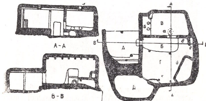
Рис. 31. План и разрез дома Расулова Рауфа, к. Хшортоб: А — айвон; Б — прихожая — кучагй; В — очажное отделение — мури; Г — чистое отделение — пасти боло; Д — кладовая — қазноқ; а — очаг — инкир; б — возвышение с двумя очагами на полу мури; в — место для стряпни — сурфахона; г — место для хранения отрубей — сабусдон; д — деревянный ларь — тавлак; е — возвышение для постельных принадлежностей.
