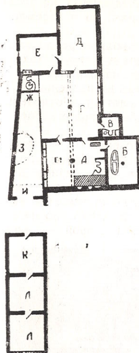
Рис. 20 Планы домов:
