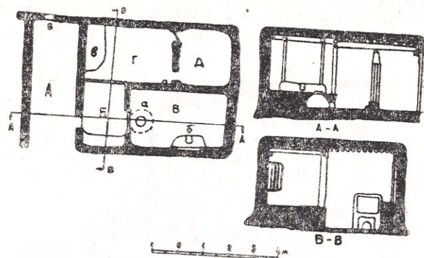
Рис. 29. План и разрез дома Расулова Бонджона, к. Хшортоб: А — веранда — айвон; Б — прихожая — кучагй; В — очажное отделение — мури; Г — чистое отделение — руи боло; Д — кладовая — қазноқ; а — очаг — инкир; б — очаг на полу мури; в — деревянный ларь — тавлак; г — свето-дымовое отверстие.
