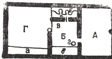
Рис. 48. План дома Икрамова Накиба, к. Вору: А — айвон ; Б — прихожая — кавшпарт ; В — очажное отделение — мур ; Г — чистое отделение — руи хона ; а — очаг для приготовления пищи — сангупоча ; б — очаг-печь для печения лепешек — оштон ; в — глинобитное возвышение для дров — суфай хезумгири ; г — яма-поглотитель — обрез ; д — возвышение для постельных принадлежностей — суфай курпатахкун .
