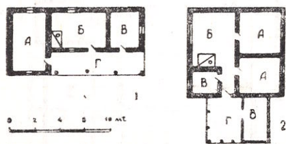
Рис. 54. Планы стандартных домов: 1 — однокомнатный дом, к. Колхозчиён; А — жилое помещение; Б — кухня; В — кладовая; Г — айвон. 2 — двухкомнатный дом, к. Колхозчиён; А — жилое помещение; Б — кухня; В — кладовая; Г — айвон.
