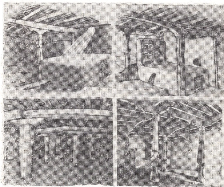
Рис. 4. Виды перекрытия: вверху слева — перекрытие традиционного жилища с одним промежуточным прогоном, к. Сабах; вверху справа — перекрытие традиционного жилища с двумя промежуточными прогонами, к. Ро.; внизу слева — перекрытие старой мечети с несколькими промежуточными прогонами, поддерживаемыми колоннами, к. Рог; внизу справа — перекрытие мечети с четырьмя колоннами, к. Мадрушкат.
