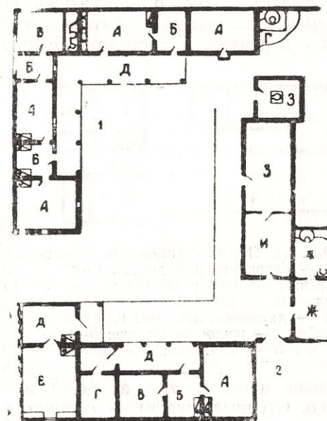
Рис. 53. Планы домов:
