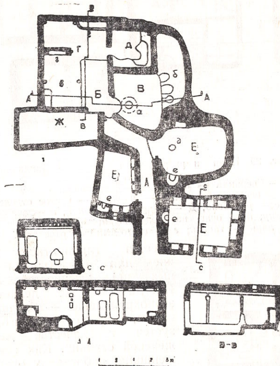
Рис. 28. План и разрез дома Хусейнова Сангина, к. Думзой: А — коридор-проход между помещениями — куча ; Б — прихожая старого жилища — куча ; В — очажное отделение — мур ; Г — чистое отделение — канна ; Д — кладовая — пистик ; Е — помещение нового вида — хучра ; Ж — помещение для топлива — сакенхона ; а — очаг, вкопанный в пол мура — инкир ; б — возвышение с очагами на полу мура; в — место для стряпни — нонгеша ; г — глиняный ларь — пича ; д — сандали; е — очаг-камин — қасаба .
