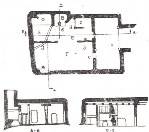
Рис. 38. План и разрез дома Бокиева Зоира, к. Ревомутк:
