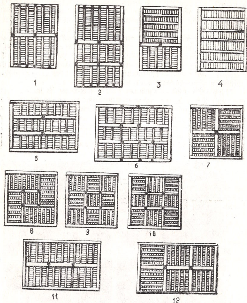
Рис. 5. Схематические изображения перекрытий: 1 — перекрытие старой конструкции с одним промежуточным прогоном, к. Сабах; 2 — то же с двумя промежуточными прогонами, к. Рог; 3 — перекрытие с элементами старой конструкции, к. Мадрушкат; 4 — перекрытие новой конструкции, к. Мадрушкат; 5 — перекрытие старой мечети, к. Сабах; 6 — то же, к. Рог; 7 — перекрытие мечети с одной колонной, к. Рог; 8—10 — перекрытия мечетей с четырьмя колоннами, отличающиеся друг от друга расположением прогонов и балок, в кишлаках Гузн, Мадрушкат и Рог; 11, 12 — перекрытия мечетей в к. Рог с двумя колоннами, отличающиеся друг от друга также расположением прогонов и балок.
