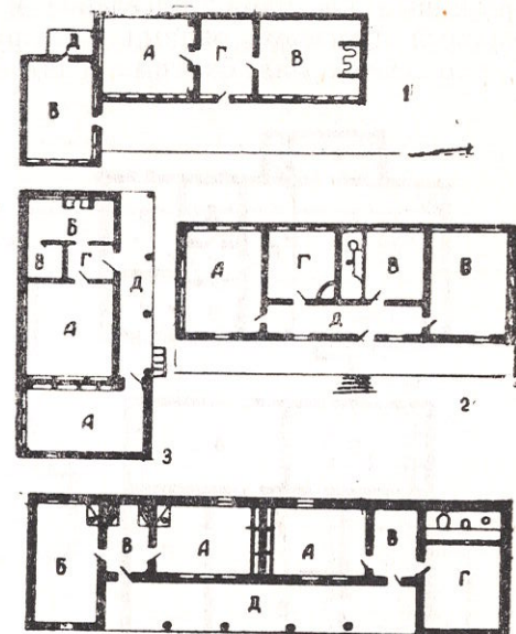
Рис. 51. Планы домов:
