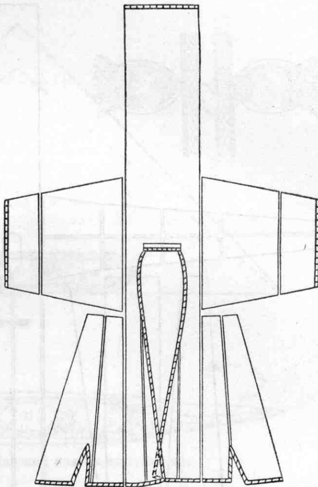
Рис. 12. Покрой калтача.
