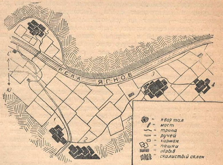
Рис. 8. Схематический план сел. Ворсоут (глазомерная съемка с высоты).
