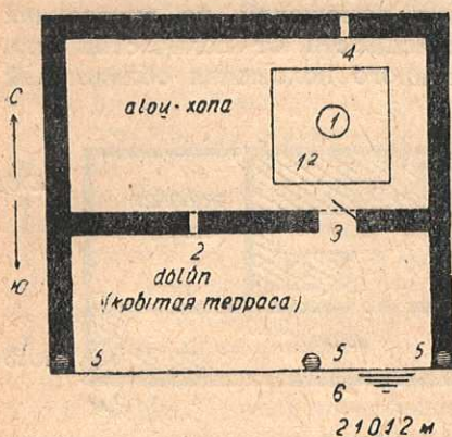
Рис. 27. План общинного дома алоу-хõпâ (ныне собственность колхоза) в сел. Оби-сафед в верхнем Варзобе. 1 — место для костра; 12 — пониженная часть пола; 2, 4 — окна; 3 — дверь; 5 — столбы, поддерживающие крышу; 6 — лестница из каменных плит.
