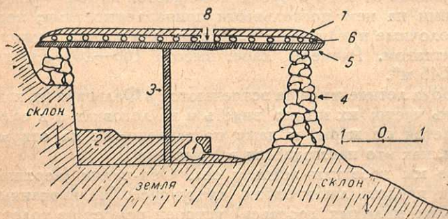
Рис. 33. Вертикальный разрез жилища на летовке. 1 — очаг; 2 — sufak; 3 — столб; 4 — стены из камня; 5 — балки; 6 — жерди; 7 — слой щебня и земли; 8 — отверстие для выхода дыма.
