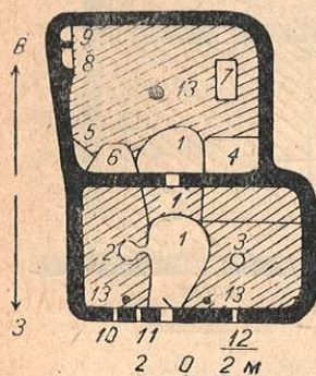
Рис. 24. Жилище Садуло Бободжона в сел. Зуман. 1 — проход; 2—3 — очаги; 4—6 — зернохранилища; 7 — переносное зернохранилище; 8—9 — ниши; 10—12 — окна; 13 — столбы.
