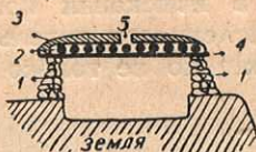
Продольный разрез
