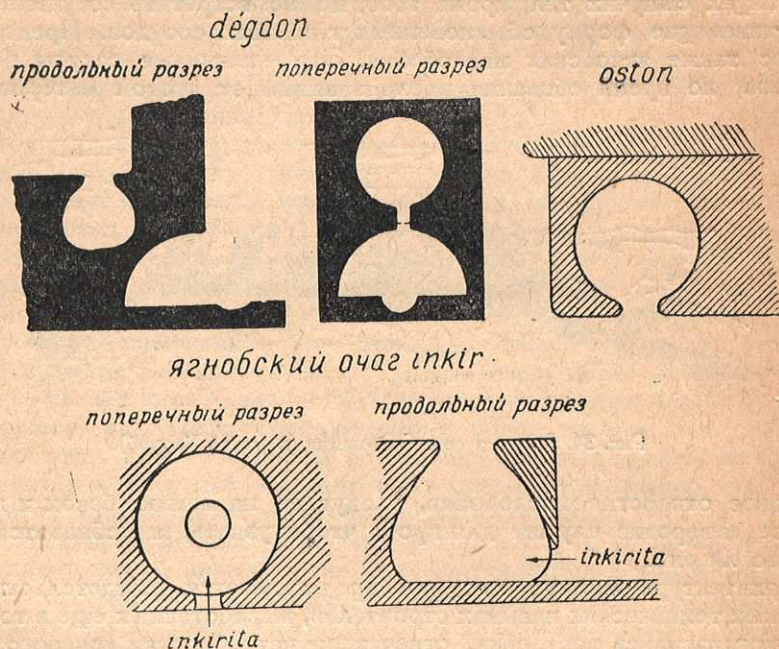
Рис. 35. Типы очагов таджиков и ягнобцев.
