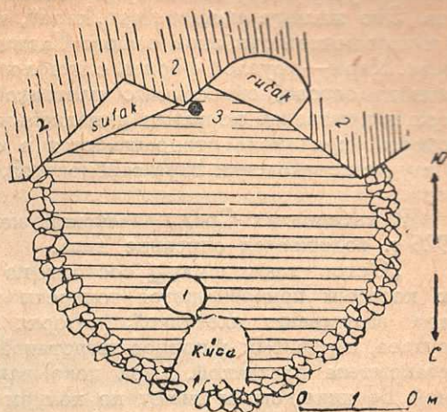
Рис. 32. План жилища на летовке Кули-миона. 1 — очаг; 2 — скала (задняя стена жилища); 3 — столб.
