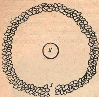
Рис. 30. План „дома для гостей“, летовка Куливорсоут. 1 — стена каменной кладки; 2 — жерди; 3 — слой щебня и земли; 4 — балки; 5 — отверстие для выхода дыма; I — проход; II — место для костра.
