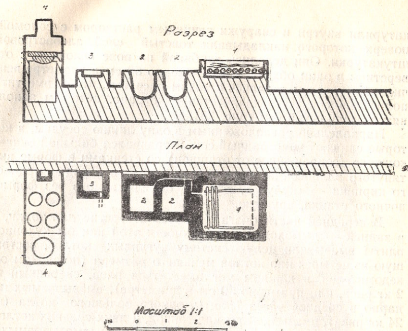
Рис. 29. 1—«чоркишт» — давяльня; 2—«чохаки» — цистерны для виноградного сока; 3—«чохаки чакка» — фильтр; 4—«оштон» — печь с вязанными котлами; 5—стена сада, к которой примыкает все сооружение.
