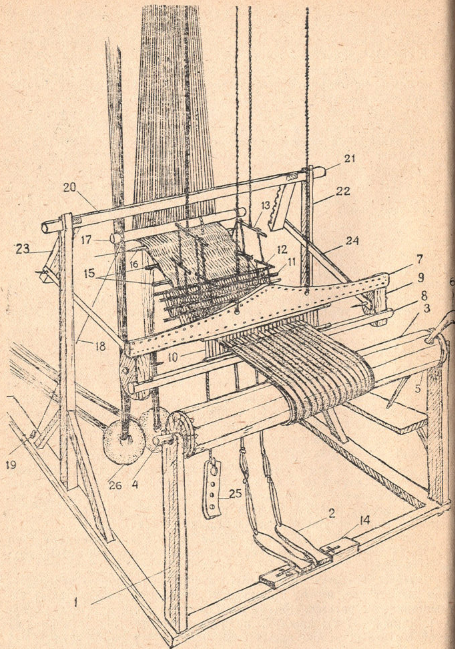
Рис. 9. Каратагский ткацкий станок — дүкони бофандаг, КП 363: 1—развилки-хачча; 2—педали-пошвол; 3—навой-навард; 4—шпы навой-гушаки навард; 5—отверстия в навое для рукоятки-чои кулоқчұб; 6—рукоятка для повертывания навой-кулоқчұб; 7—верхняя планка батана-сакаъза; 8—нижняя планка батана-тагавза; 9—соединительные бруски батана-арман; 10—гребень или бердо-тег; 11—камышинки, к которым привязаны ниточки-килк; 12—малое коромыслище ремиз-гунчишак; 13—большое коромыслище ремиз-аспак; 14—передняя доска рамы, на которой монтируется станок-кундай пошвол; 15—тонкие шпиртели-разделители-бодкамиш; 16—толстый ширитель-узлук; 17—короткий оттягиватель основы-синачұб; 18—веревки оттягивателя-банди синачұб; 19—колышки для привязывания веревок оттягивателя-мехи синачұб; 20—длинный оттягиватель-паткол; 21—шпы на концах длинного оттягивателя-турми паткол; 22—стойки для длинного оттягивателя-хаччи паткол; 23—брусочки длинного оттягивателя-оринчак; 24—планки, соединяющие бруски длинного оттягивателя с рамой-батаном-шамшерак; 25—малое грузило-олтношук; 26—большое грузило-борсанг
