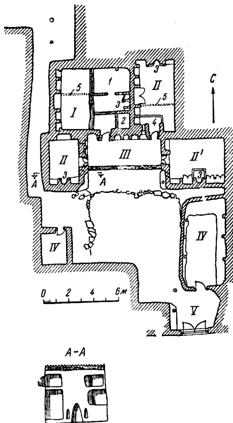
Рис. 9. Дом в Сарытаге. План и разрез худжры: I — хона; II — худжра; III — айван; IV — огул (помещение для овец); V — дарваза (крытые ворота); 1 — тахтакона; 2 — ташнаб; (водослив); 3 — оштон; 4 — кавш-каши, 5 — сим-каши
