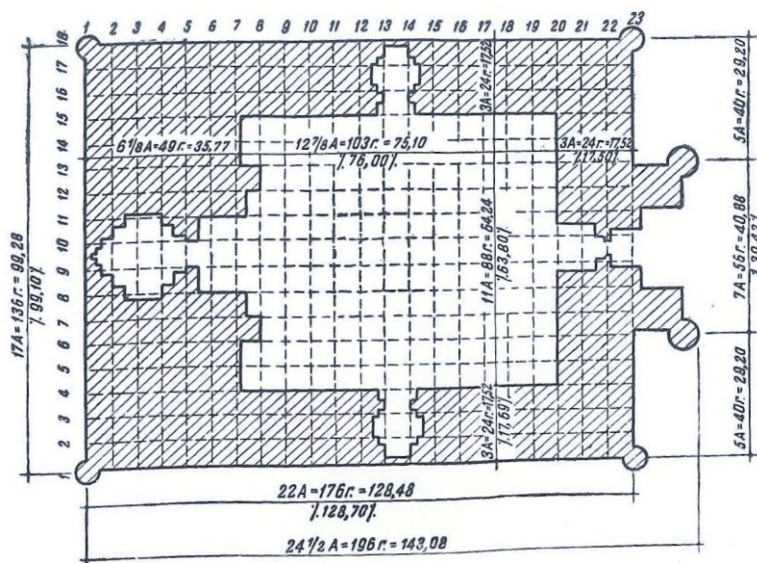
Рис. 82. Биби-ханым. Анализ построения плана всего комплекса мечети.
