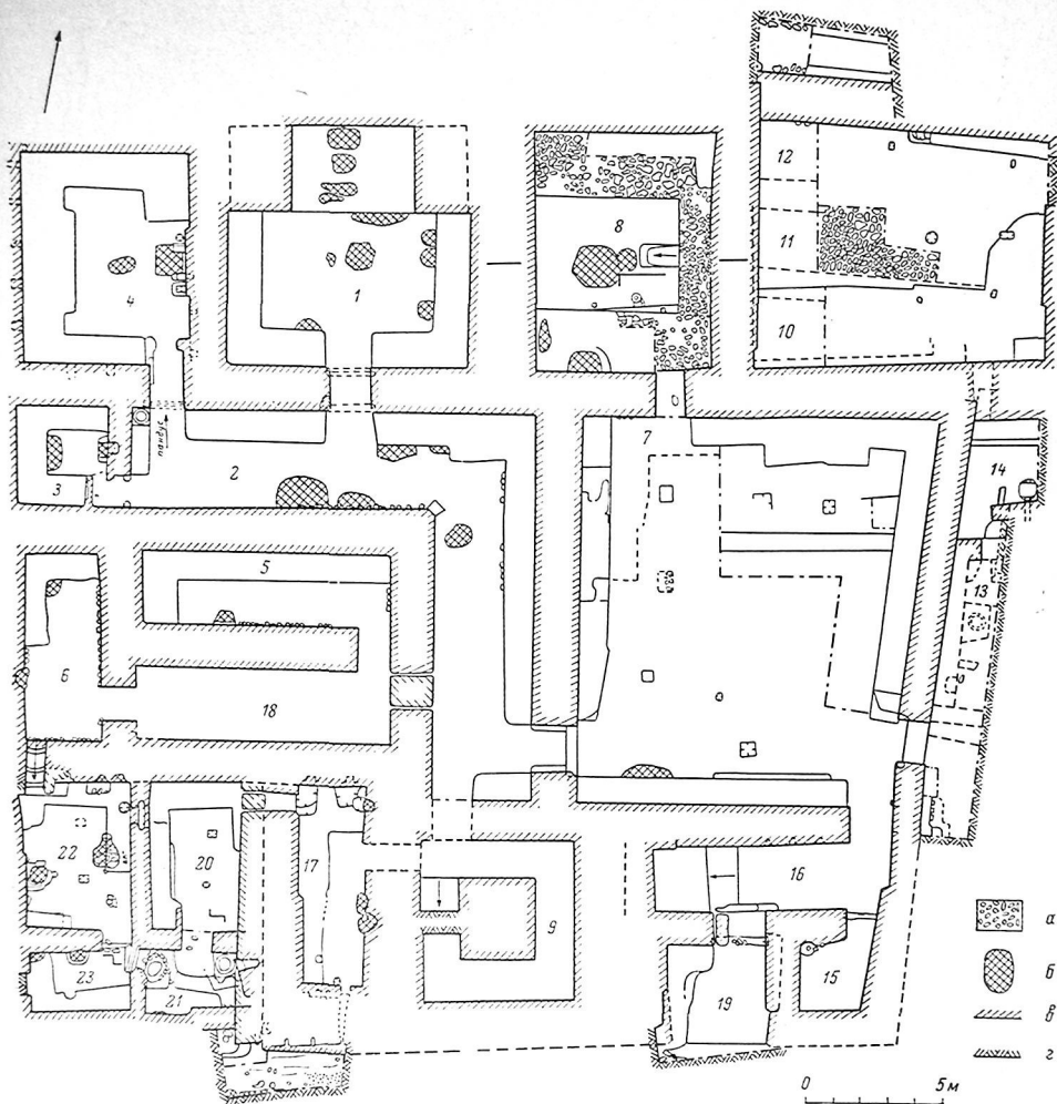
Рис. 25. Пейджикент. Объект XXI. План.
