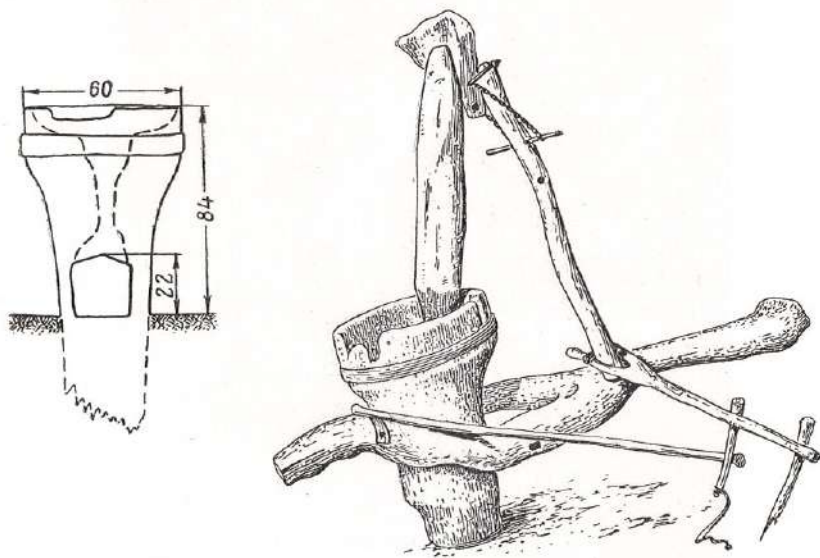
Рис. 6. Маслодельня «джугаза» семиреченских уйгуров
