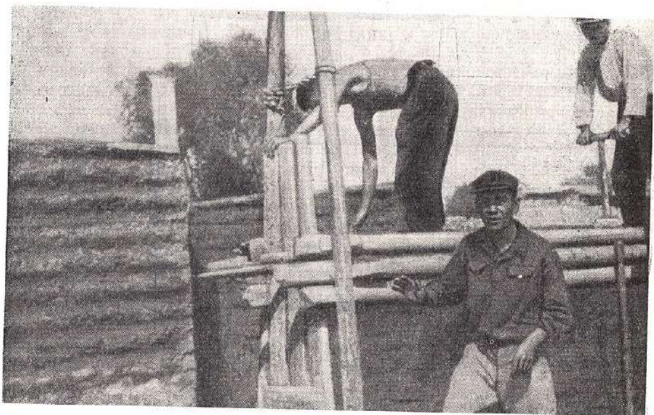
Рис. 16. Возведение стен способом «сокма». Сел. Б. Аксу, Уйгурский р-н Алма-Атинской обл.
