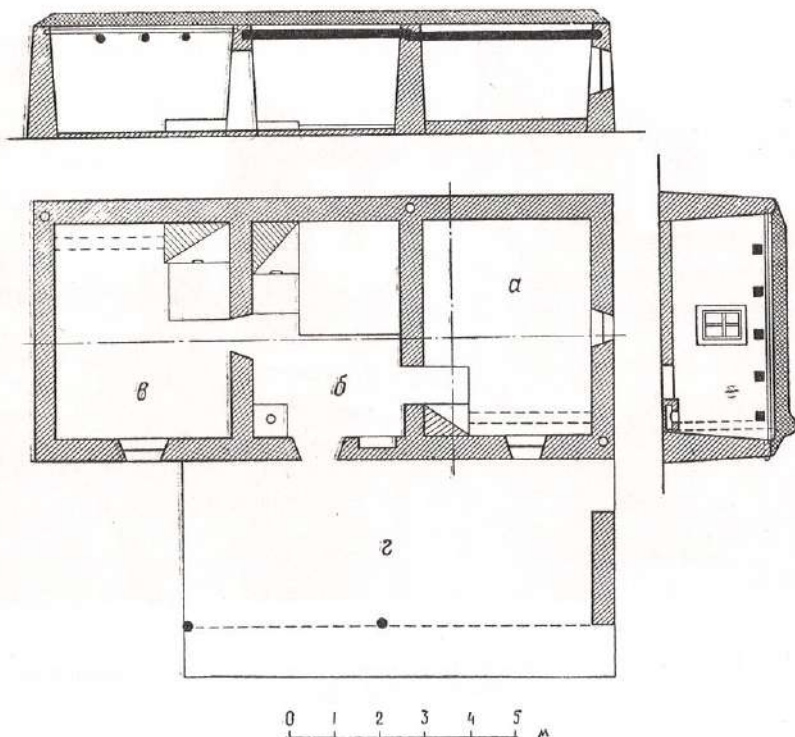
Рис. 15. План дома Ошрапа Осипова:
