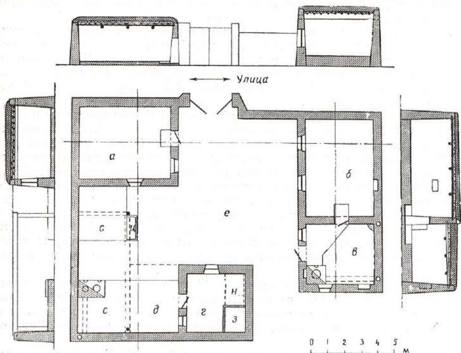
Рис. 14. План дома Ушура Аметова:
