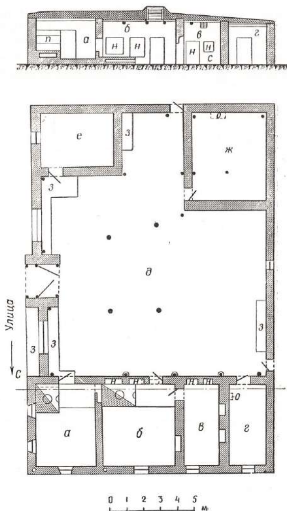
Рис. 12. План усадьбы семиреченских уйгуров: (1-й тип):
