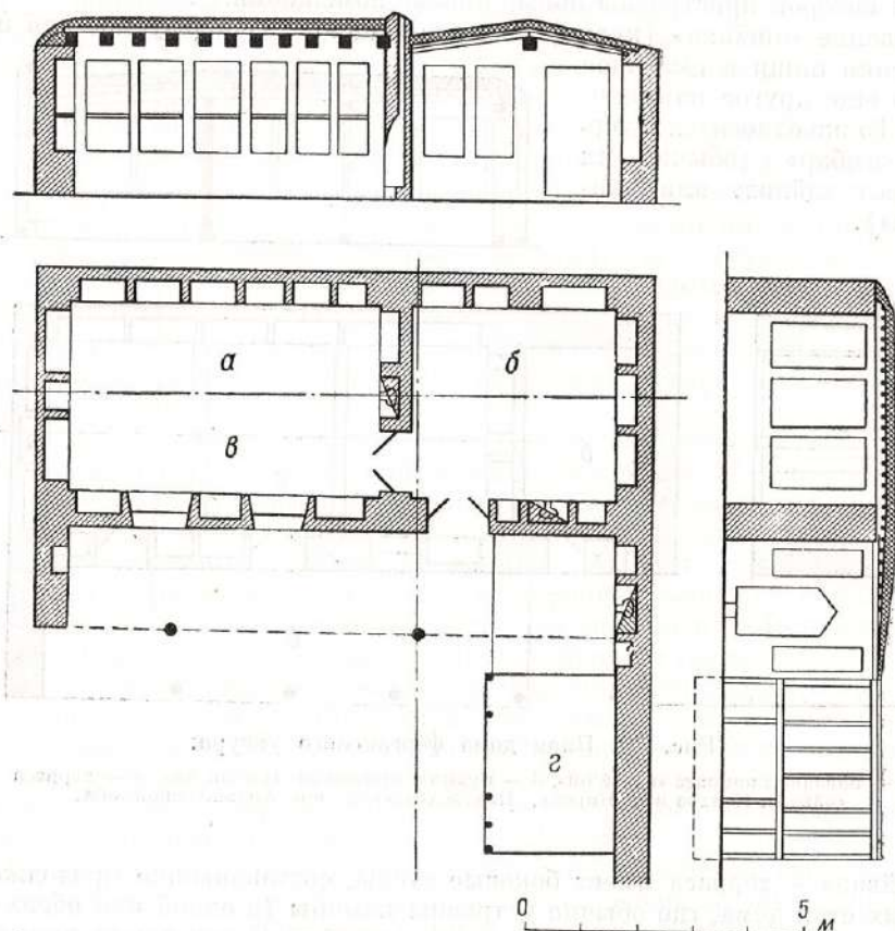
Рис. 24. План дома ферганских уйгуров:
