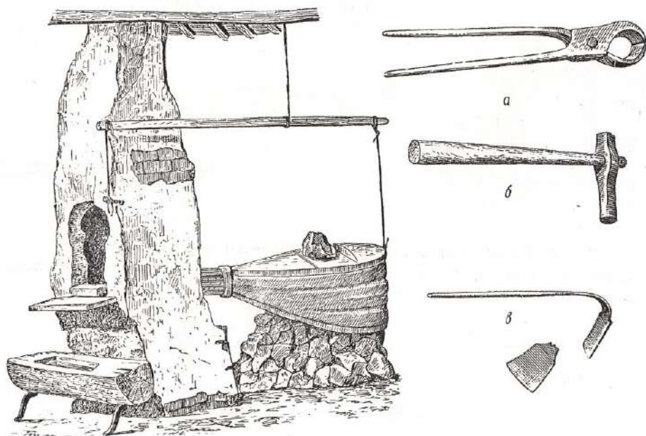
Рис. 8. Кузнечный горн семиреchenских уйгуров и инструментарий кузнеца:
