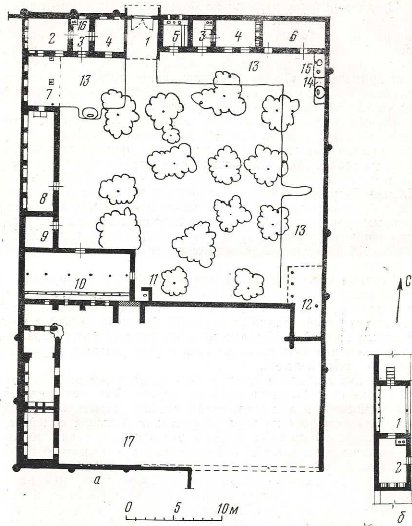
План усадьбы рабат в кишлаке Джанга-Карасыйрак, принадлежавшей в прошлом богатому крестьянину Ахматбаю:
