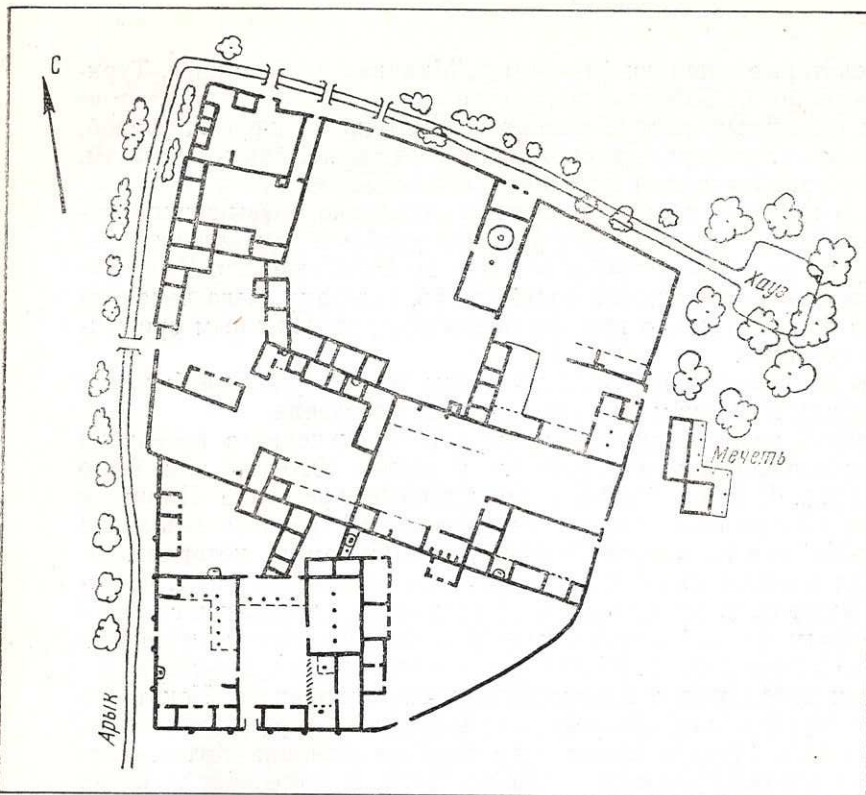
План оставшейся части кишлака Дунг до полной реконструкции (черт. Ю. В. Стеблюка)
