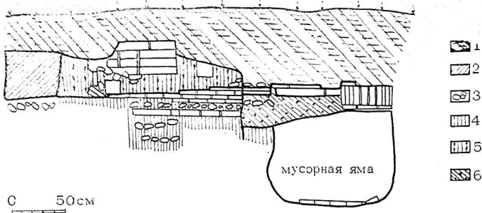
Рис. 82. Разрез в южной части шахристана:
