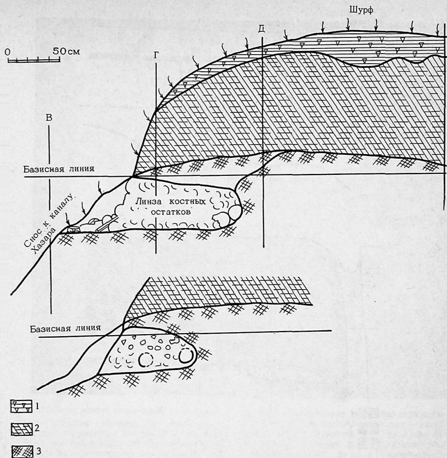
Рис. 75. Разрез через оссуарно-костные захоронения Ишм-1:
