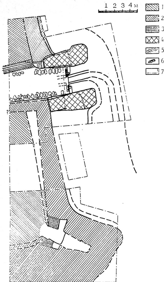
Рис. 28. Цитадель. Угловой бастион и ворота:
