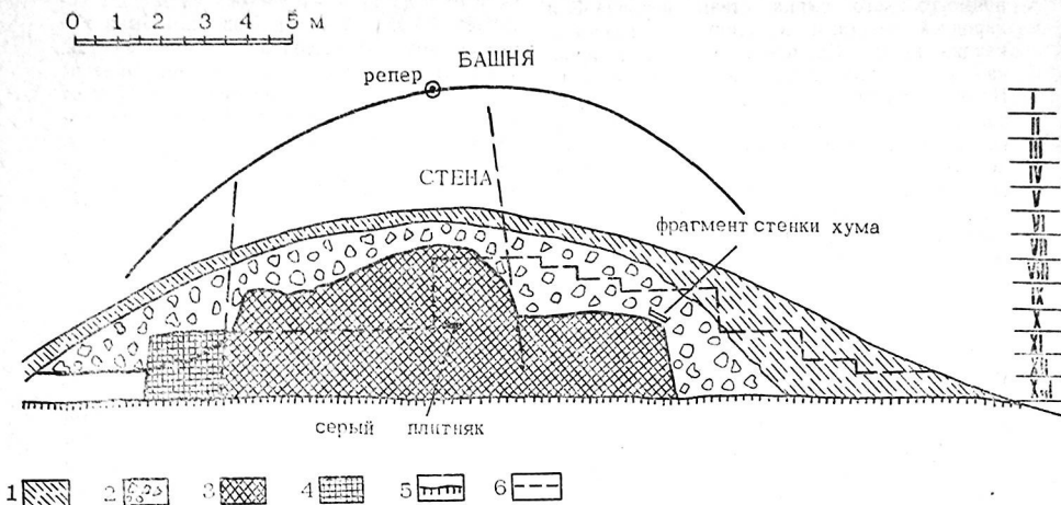
Рис. 29. Разрез стены Шахристана-I:
