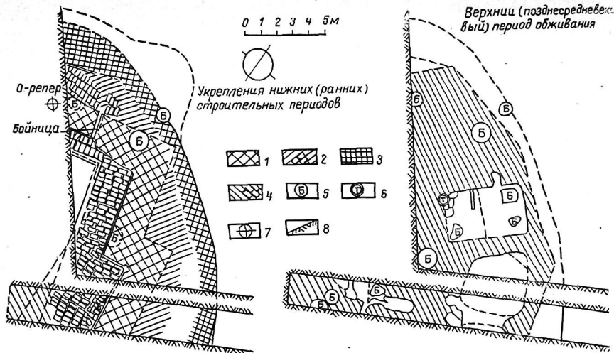
Рис. 24. Кургантепе. Цитадель. План. Раскоп 1. Разрез 1.
