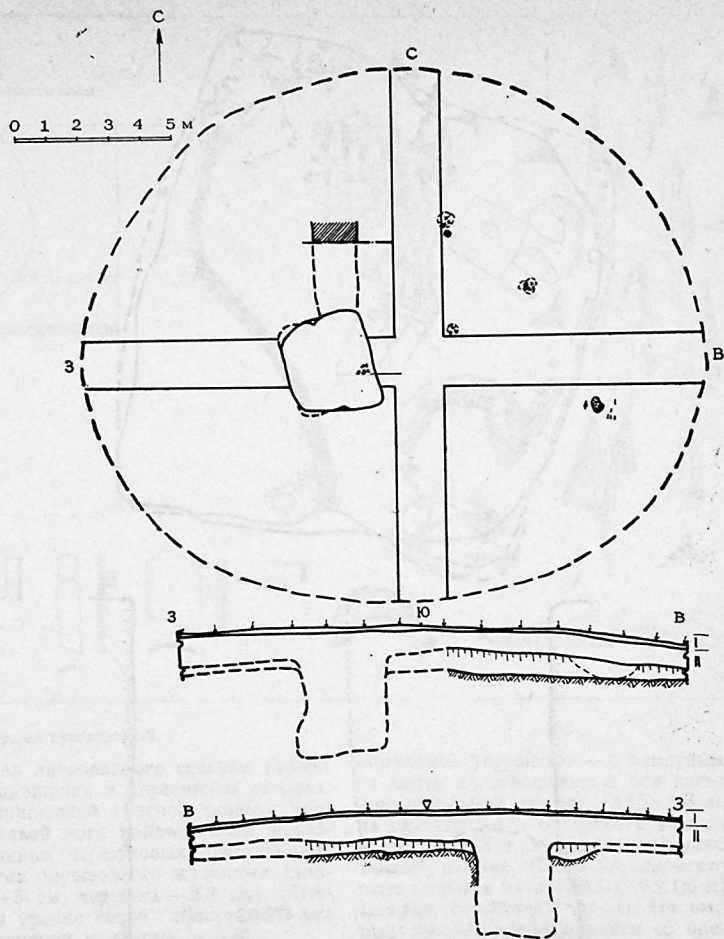
Рис. 59. Кургan Кт-9. План верхнего горизонта и разрезы.
