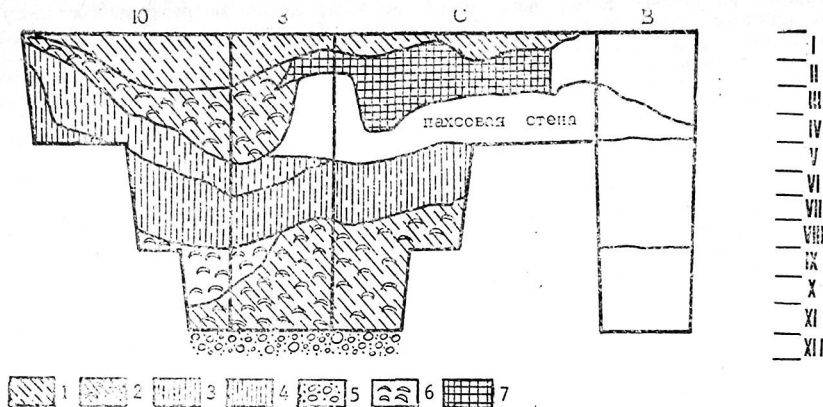
Рис. 30. Стратиграфический шурф в Шахристани-1:
