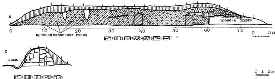
Рис. 35. А — Разрез у дороги через большой южный холм Шахристана-II; Б — разрез стены Шахристана-II. А: 1 — дерновый слой; 2 — оплыв пахсы; 3 — пахса; 4 — глина; 5 —
