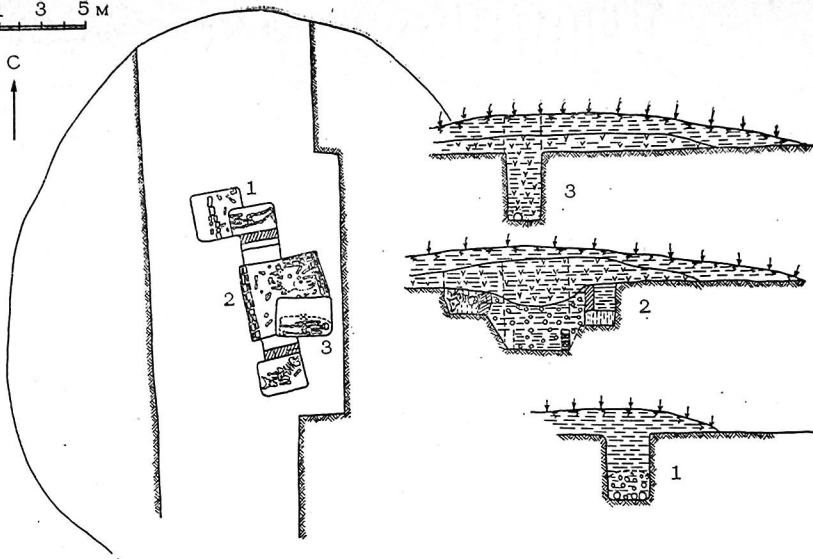
Рис. 53. Курган Кт-1. План и разрезы погребений.
