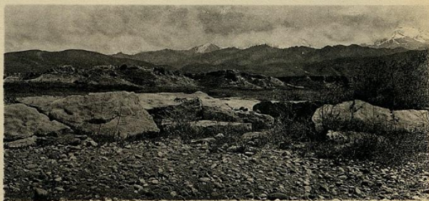
Южный берегъ оз. Исыкъ-куль около устья р. Барскаунъ. Озерная терраса и аркозовые песчаники ея нижняго горизонта.
