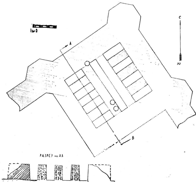
План замкового сооружения. Объект I. Третий строительный горизонт.
