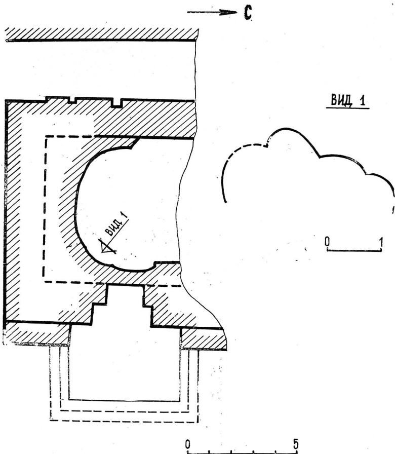
Раскоп VII. Буддийский храм. План святилища по верхнему ярусу. Раскопки 1980 г. Контур лицевой арки трюмпа.
