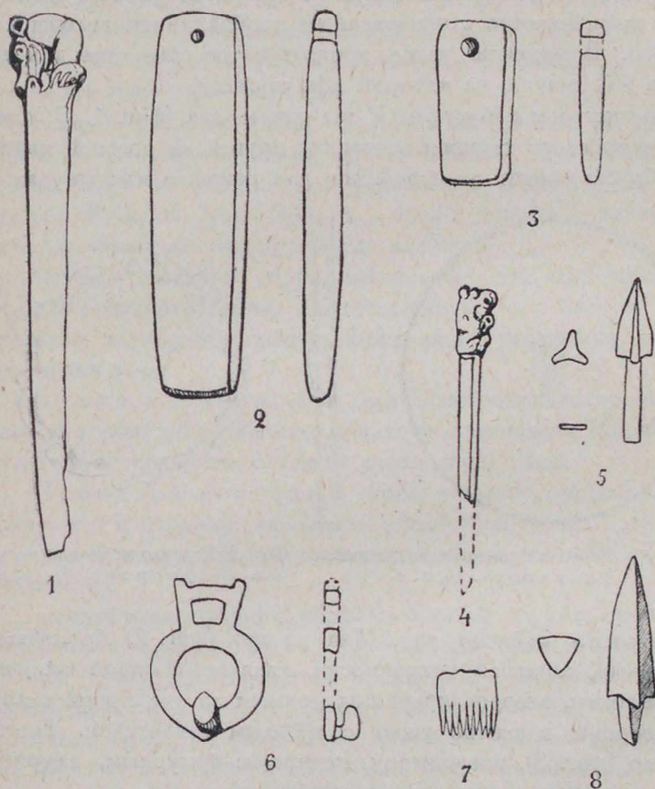
Фиг. 1. Предметы из раскопок А д р и а н о в а в Бухтарминском уезде. 1 — нож бронзовый; 2 и 3 — бруски точильные; 4 — шильце костяное; 5 — наконечник стрелы бронзовый; 6 — пряжка бронзовая; 7 — гребень костяной; 8 — наконечник стрелы костяной. 1/2 н. в.
