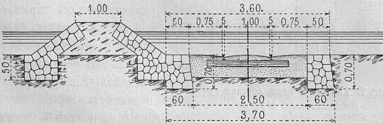
Фиг. 4. Нормальный профиль затопляемаго пути (линія Суссъ-Кайруанъ).
