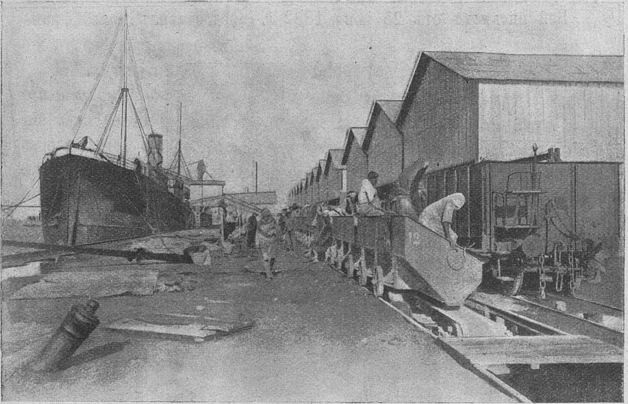
Фиг. 13. Набережная для нагрузки фосфатовъ въ портъ Сфаксъ.
