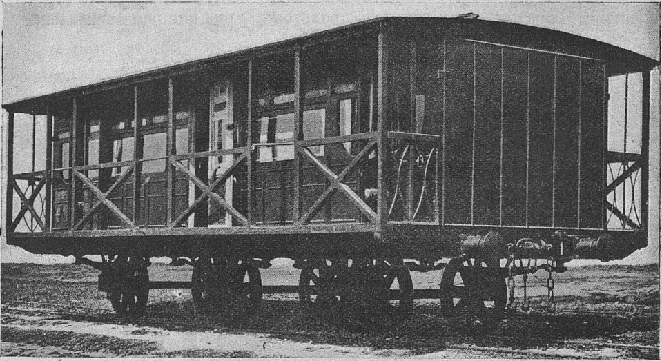
Фиг. 11. Вагонъ-салонъ тунисскаго бей, на сѣти Тунисъ—Гулеттъ-Марса.
