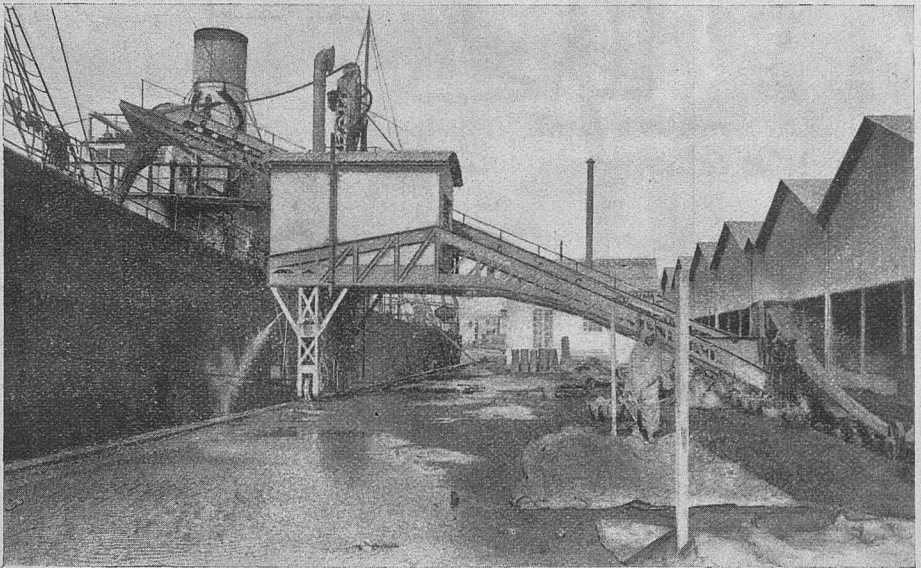
Фиг. 14. Автоматическая перегрузка фосфатовъ изъ вагоновъ на пароходы въ портъ Сфаксъ.
