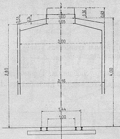
Фиг. 7. Габаритъ подв. состава тунисскихъ жел. дорогъ.
