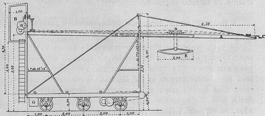
Фиг. 16. Схема снаряда для механической укладки верхняго строенія.
