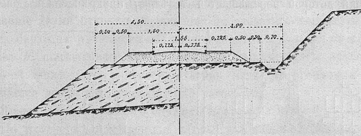
Фиг. 2. Нормальный поперечный профиль тунисских ширококолейных желѣзныхъ дорогъ.
