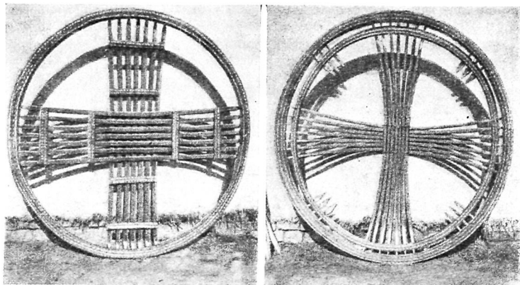
Рис. 21. Шангараки a — казахской юрты; б — каракалпакской юрты
