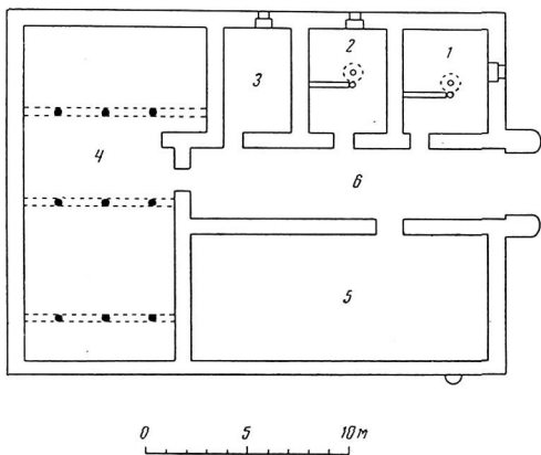
Рис. 25. План усадьбы Сундетбая (конец XIX в.) 1, 2 — жилые комнаты; 3 — данхана; 4, 5 — сейсхана; 6 — дализ
