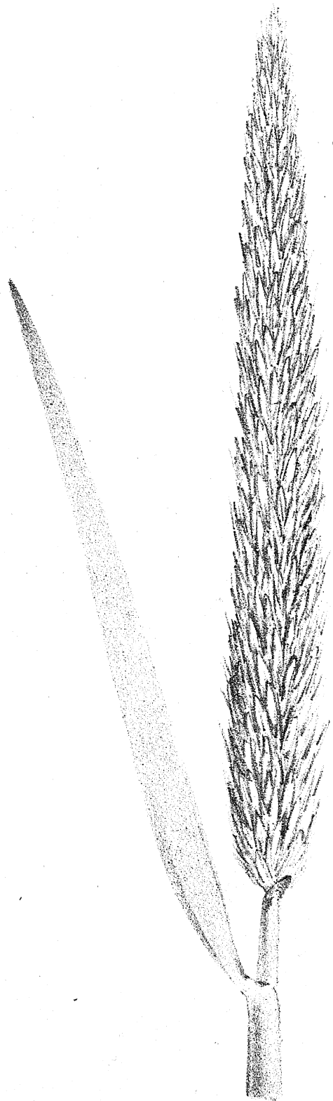
Elymus sabulosus.
