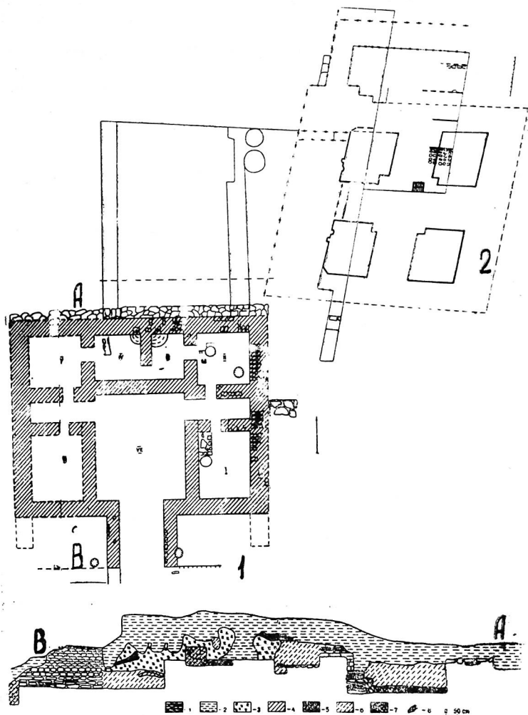
Рис. 30. План и разрез отдельно стоящего здания 1: 1 — кладка кирпича; 2 — за- хоронения; 3 — рушенный кирпич; 4 — глина; 5 — глина с галькой; 6 — зольник; 7 — пахса; 8 — очаг; 2 — план культового сооружения.
