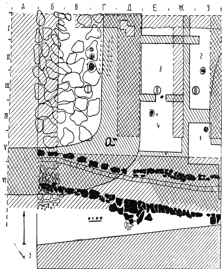
Рис. 6. План жилых помещений юго-восточной части шахристана.
