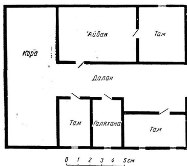
Рис. 6. План жилого дома. Кипчакский район
