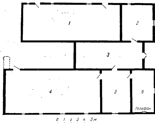
Рис. 3. План здания правления колхоза им. Ленина
