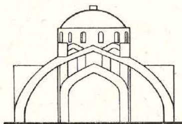
Купольная система на пересекающихся арках: а) Токи-Саррофон (XVI в.); б) Хонако Бахаведдин (XVI в.); в) Хонако при медресе Миракон (XVI в.).
