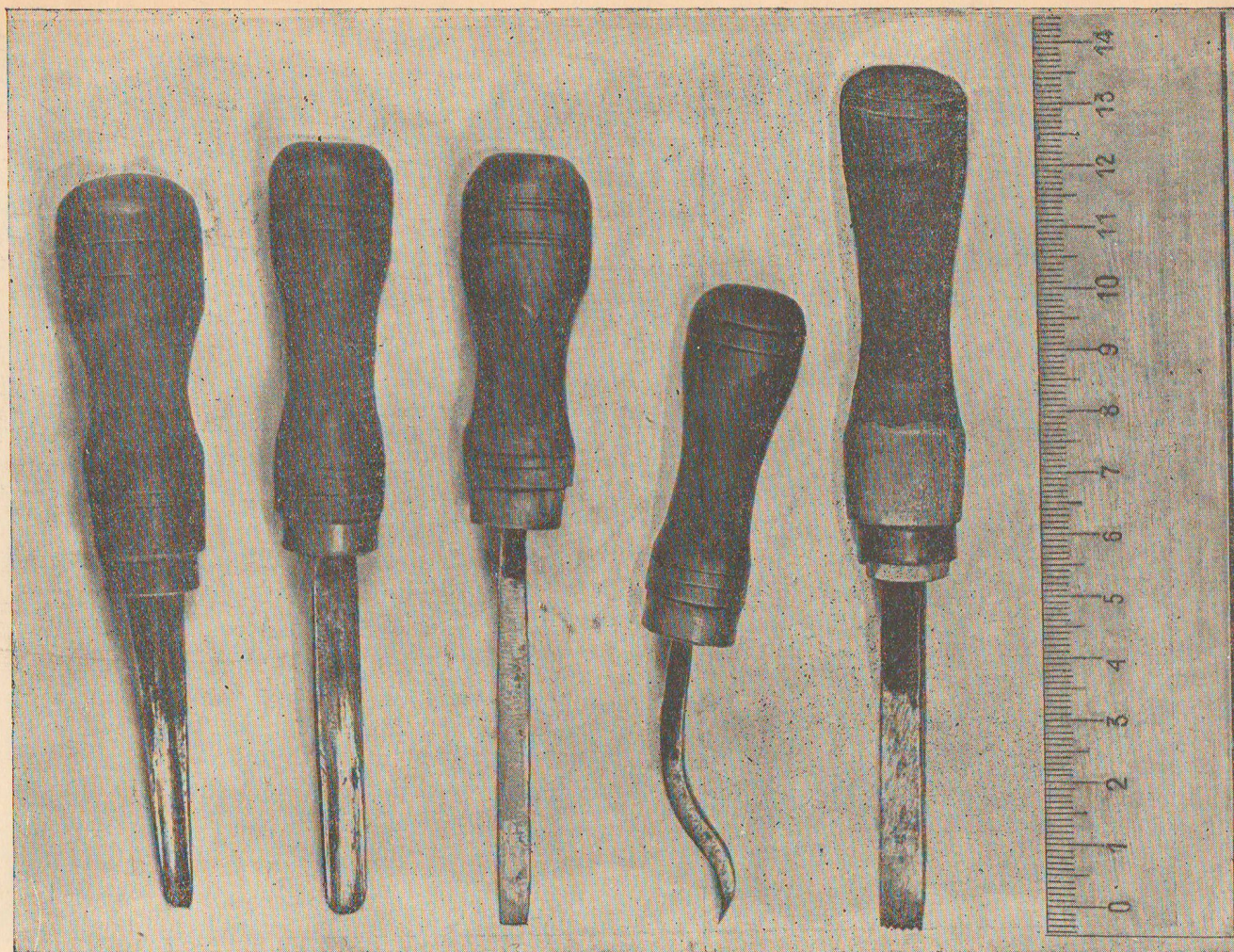
3. Инструменты для резьбы по дереву (слева направо): „нау искона“—инструмент с сильно закругленным рзцом. „балик сирт“—инструмент со слегка выгнутым резцом, „тогри искона“— инструмент с прямым резцом, „замин калям“—для выборки фона, „гурзи“—для обработки фона мелким наколом.
