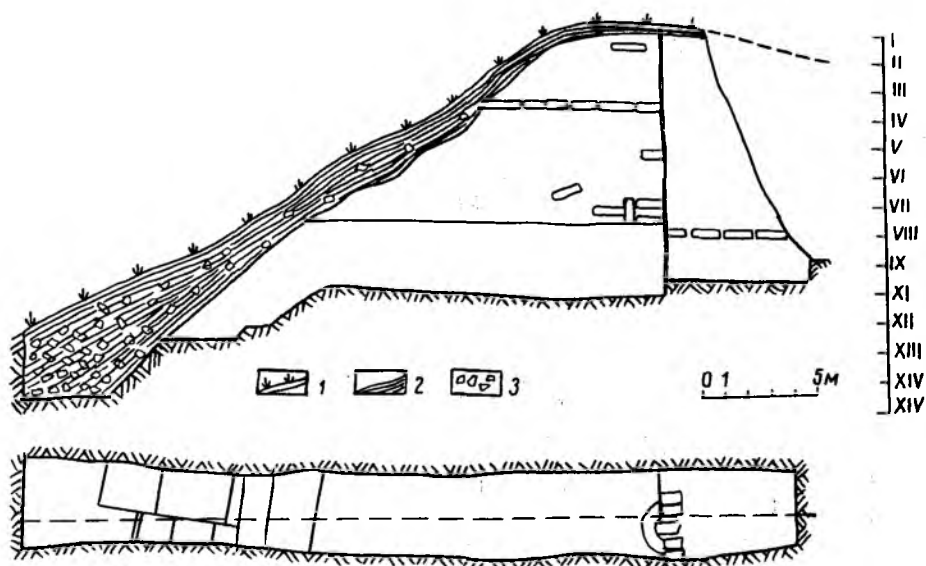
Рис. 49. Поперечный разрез кладки восточной стены сооружения центрального холма храмового комплекса на Р-1: 1 — дерн; 2 — слой оплыва; 3 — обломки пахсовой кладки.
