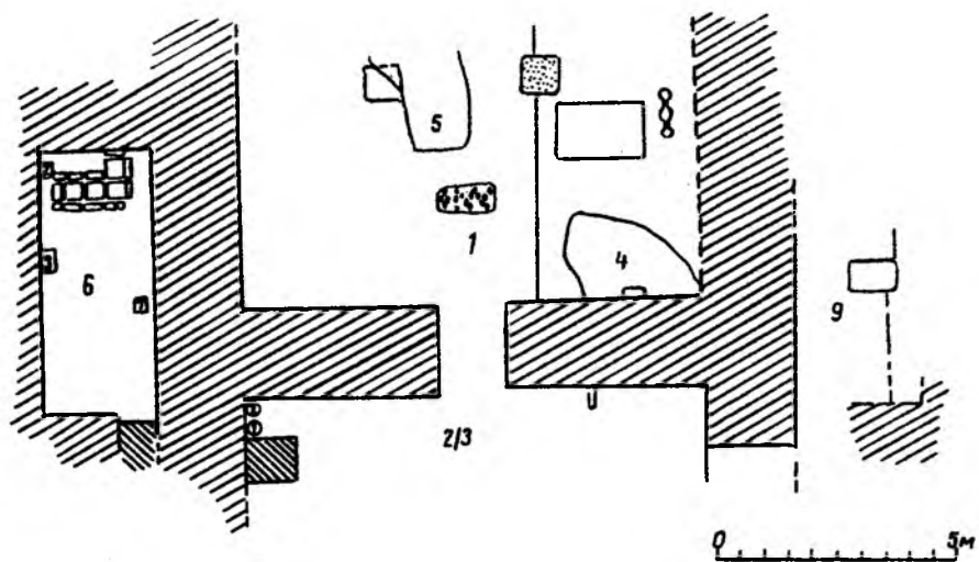
Рис. 62. Общий план мавзолея Еркургана (Р-4).
