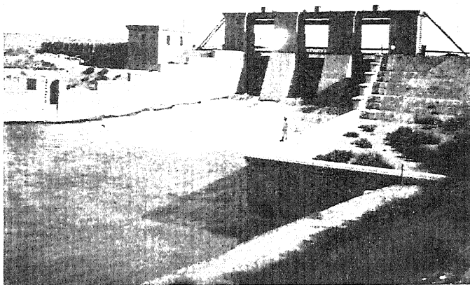
Рис. 2. Султанбентская плотина въ Государевомъ имѣніи на р. Мургабъ со стороны водослива.
