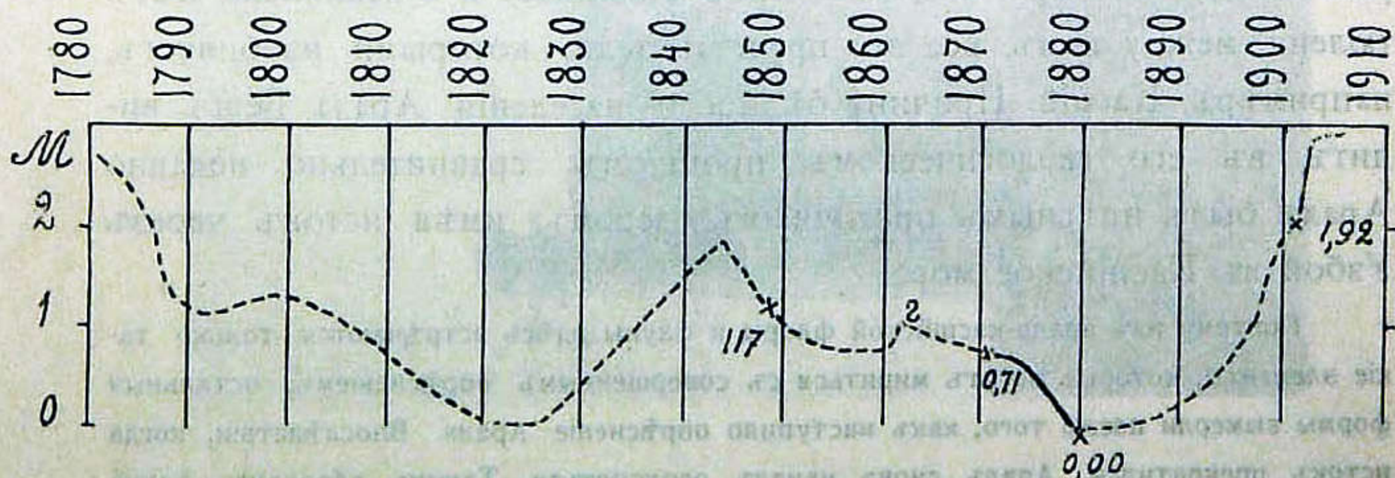
Колебанія уровня Аральскаго моря.
