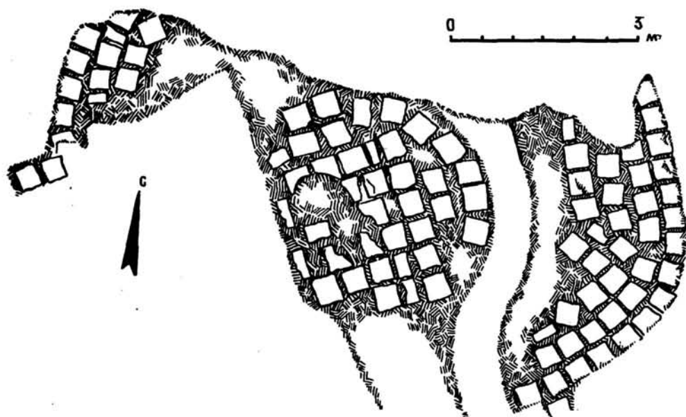
Рис. 6. Городище Тепан-шах. Раскоп 3. План.
