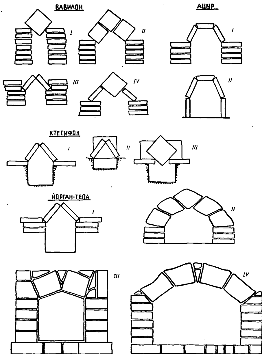
Рис. 23. Типы западнопарфянских погребальных склепов.
