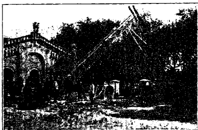
Фиг. 42. Установка столбовъ воздушной линіи высокаго напряженія для электропередачи.
