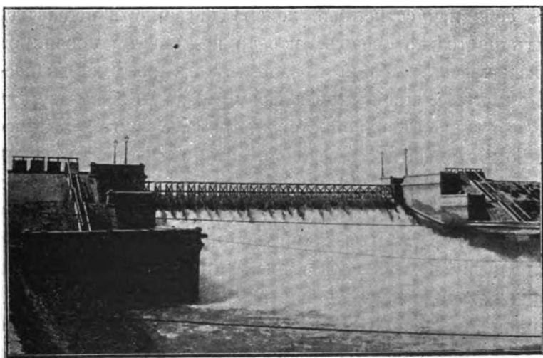
Хидыкушская плотина.
