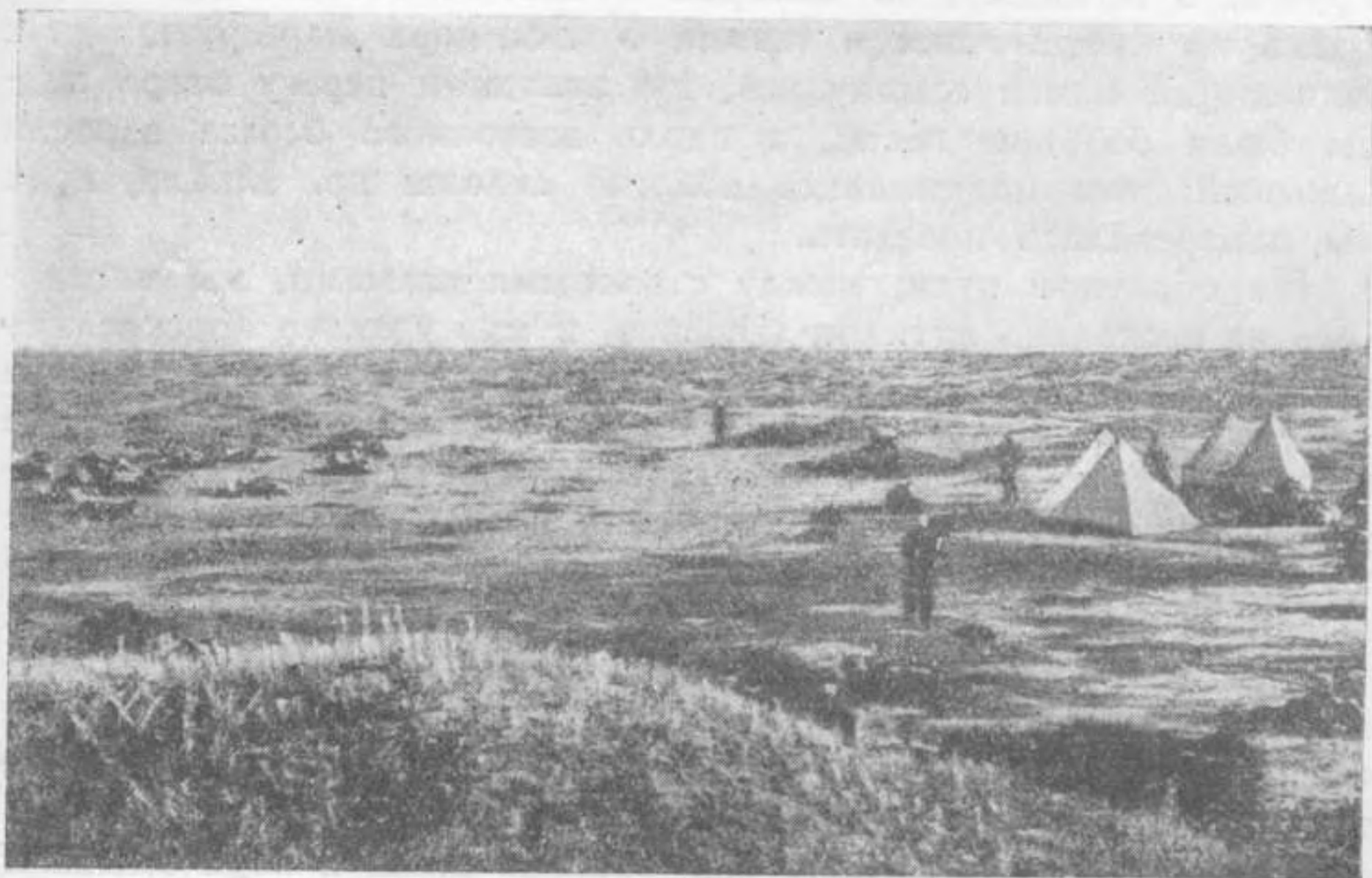
Рис. 30. Хармыковский тип кучевых песков на дне одной из впадин Центральной Азии (фото П. К. Козлова)
