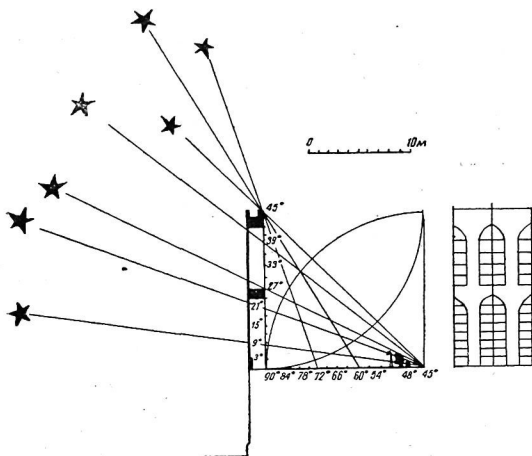
Рис. 5. Методы наблюдения светил в четвертных секторах II и III ярусов.
