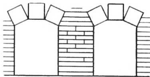
Рис. 14. Устройство забулки сводов галереи
