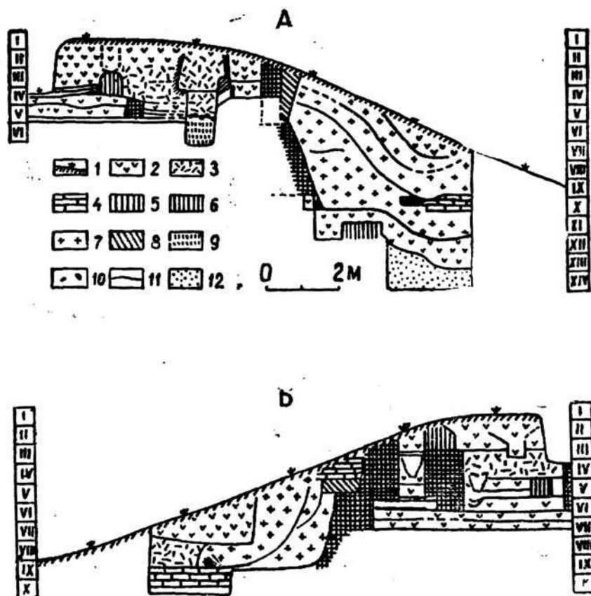
Рис. 14. Холм № 7. Боковые стенки стратиграфического раскопа. А — западная стенка, Б — восточная: 1 — «пушонка»; 2 — рылый культурный слой; 3 — завал; 4 — сырец; 5-6 — стены; 7-8 — пахса; 9 — пепел; 10 — камни; 11 — зольные прослойки и уровни полов; 12 — песок.
