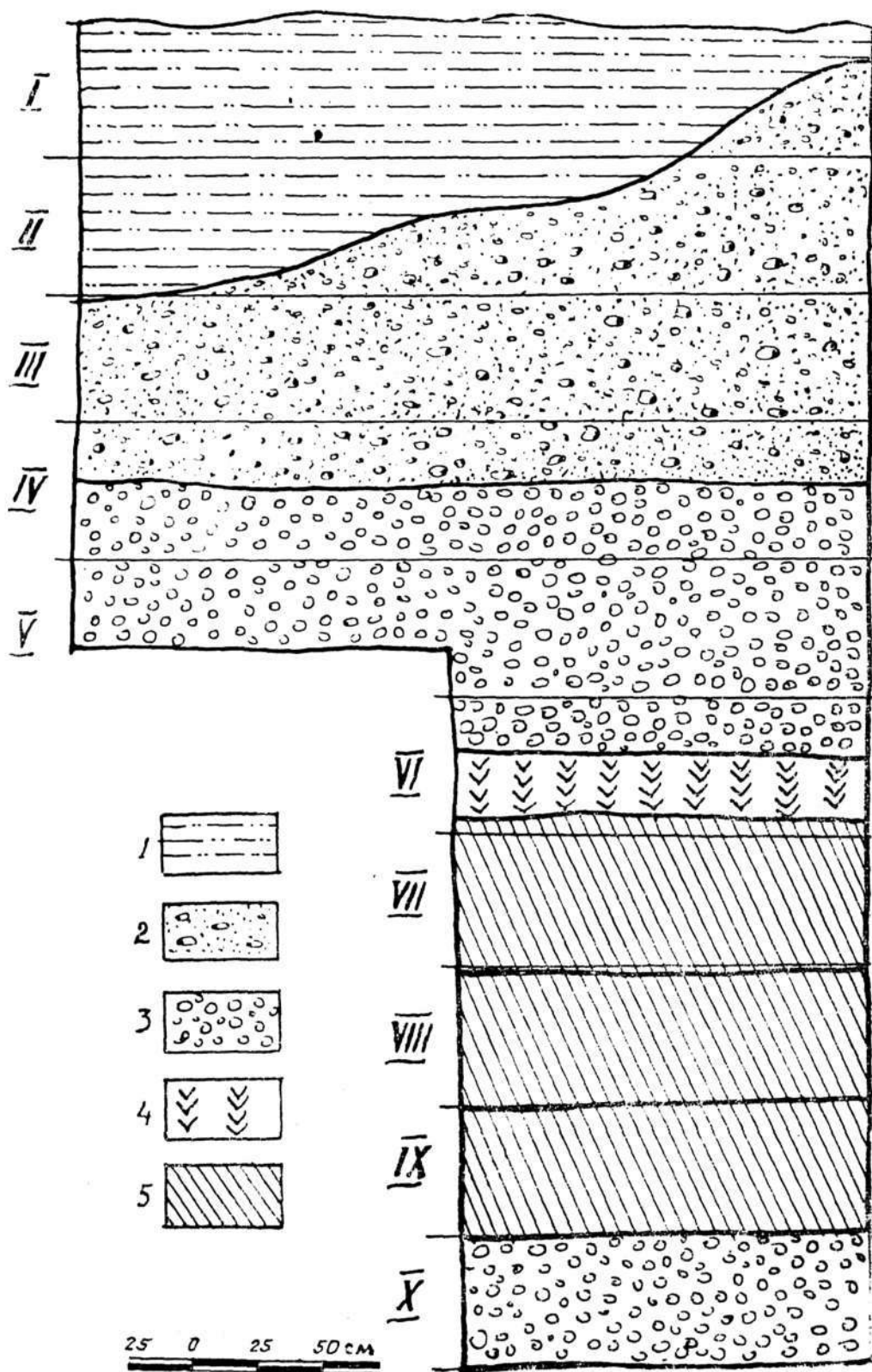
Рис. 49. Городище Калан Кяхкаха III. Шурф № 1. Разрез восточной стенки: I—современная мусорная яма; 2—желто-серый лёсс с галькой; 3—галечник; 4—жел- тый глинистый лёсс. 5—серовато-желтый слой с прослойкой из костей и керамики.
