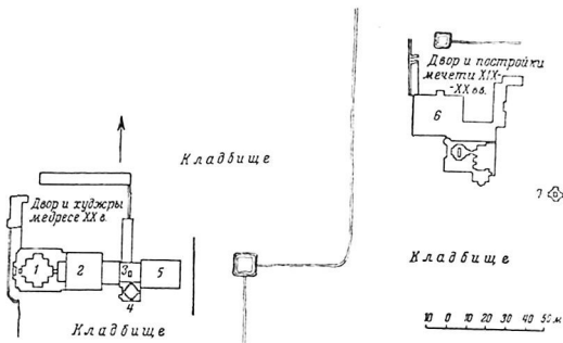
Генеральный план сооружений в юго-западной части Шахрисаяба: 1—Кул-Гумбаз, 2—мечеть XX века, 3—мазар шейха Куляля, 4—так наз. „Гумбаз-и-Се'аядан“, 5—мечеть XVI—XVII веков, 6—так наз. „Хазрет-и-Имам“, 7—так наз. „Склеп Джехангира“.
