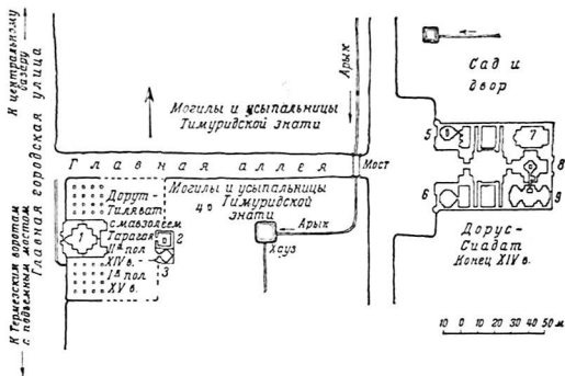
Реконструкция плана ансамбля зданий XIV—XV веков в Шахрисаябе:
