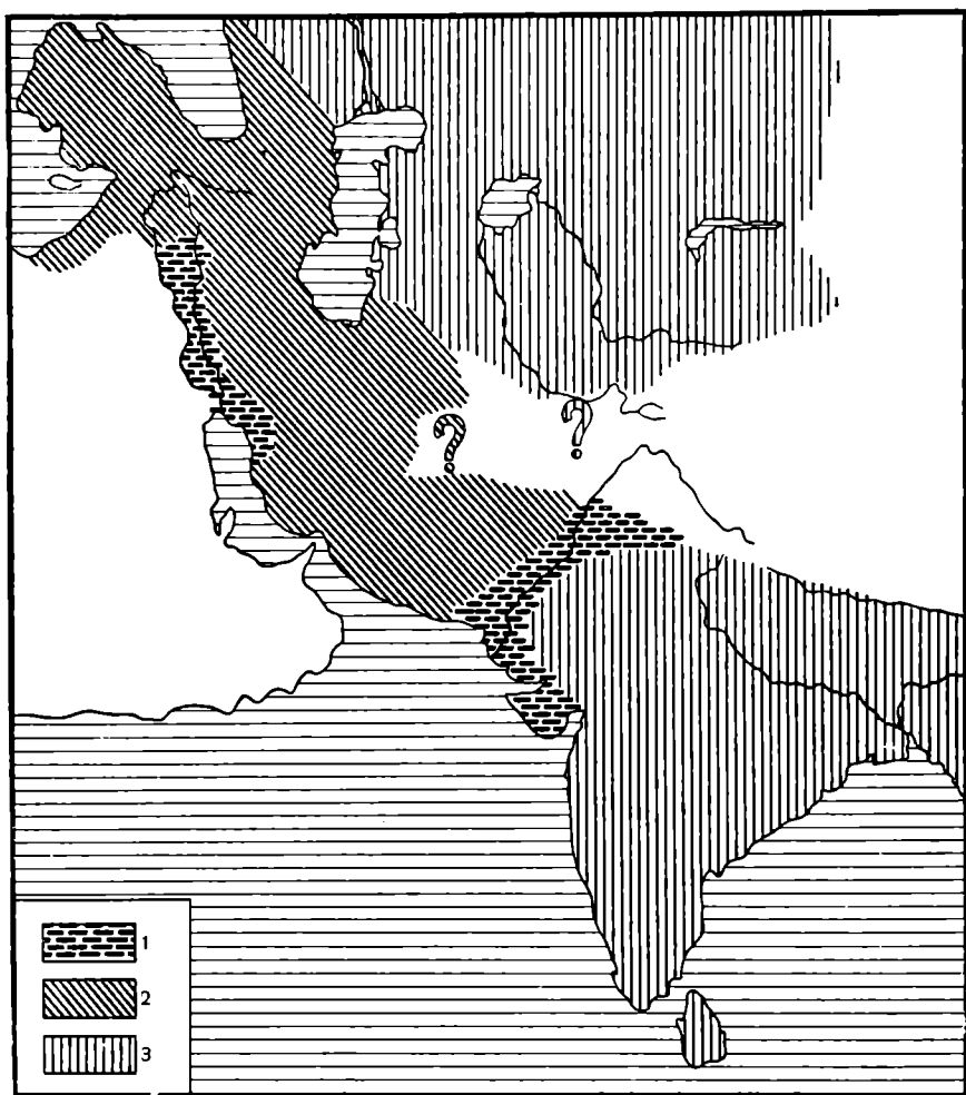
Рис. 2. Юго-Западная Азия в IV—III тысячелетиях до н. э.
