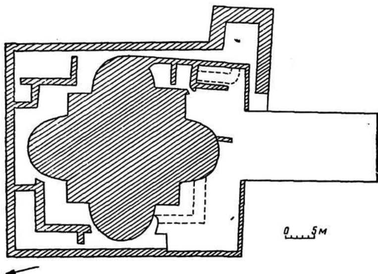
Рис. 33. План Сеталака-I в конце II строительного периода
