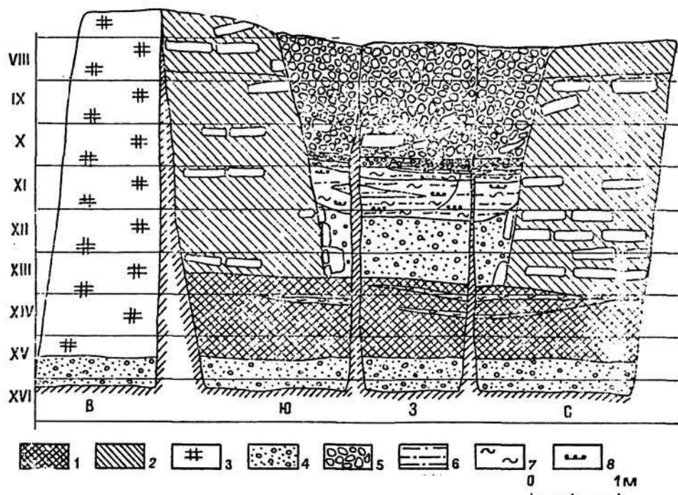
Рис. 28. Развертка стенок стратиграфического шурфа у северо-западного угла здания I строительного периода:
