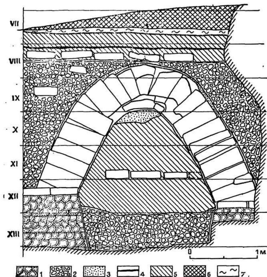
Рис. 31. Разрез свода помещения 9:
