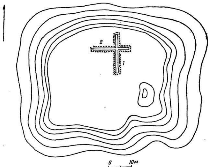
Рис. 20. Нортэпа. Общий план:
