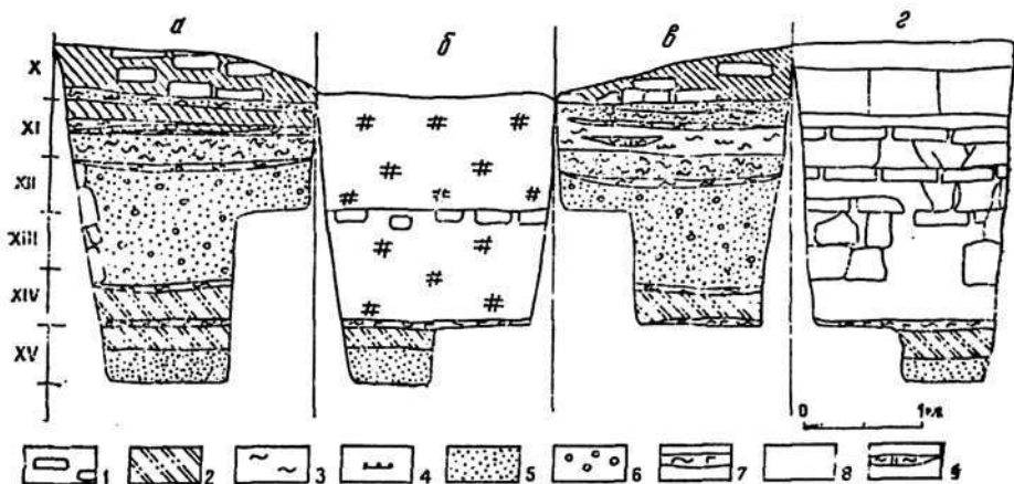
Рис. 27. Развертка западной (а), северной (б), восточной (в) и южной (г) стен шурфа на северном склоне Сеталака-I второго строительного периода:
