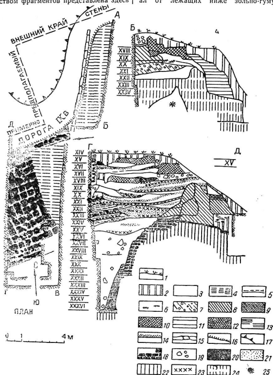
Рис. 1. Разрезы западного и северного отрезков восточной стенки раскопа 41/XVI и план городской стены IV—III вв. до н. э.
