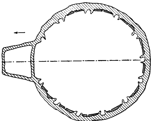
Рис. 1. План гончарной печи
