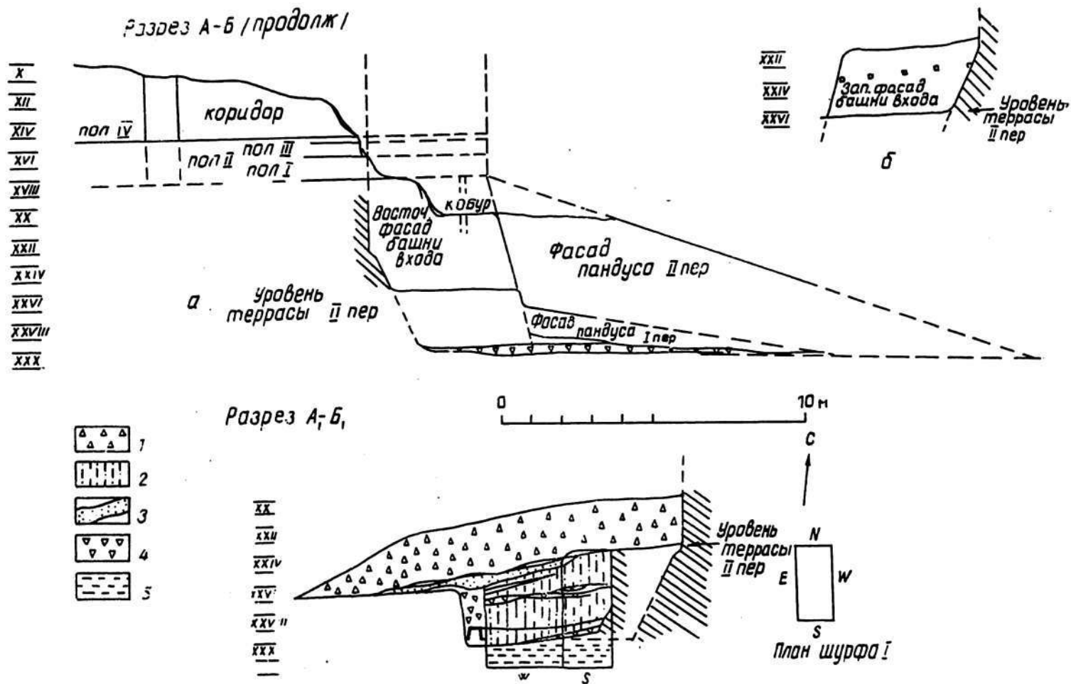
Рис. 43. Бинкат. Актёпа Юнусабадское. Разрез у входной башни: 1 — слой сырого завала; 2 — слой средней плотности; 3 — зольная прослойка; 4 — гумус; 5 — лессовый материк.
