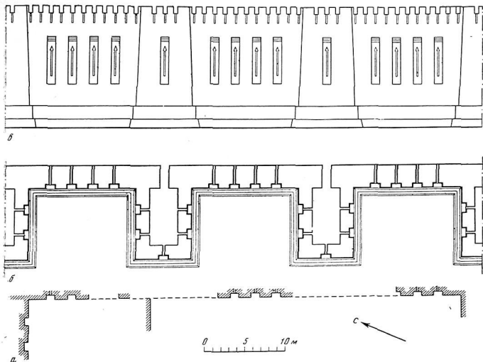
Рис. 35. Крепостная стена периода I. Фрагмент фасада а — участок зачистки внешнего контура стены на склоне заднего вала (между первой и четвертой башнями); б — план этого участка (реконструкция); в — фасад (реконструкция)
