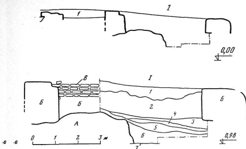
Рис. 27. Разрезы I—I через наслоения между зданием I и древней стеной, ограничивавшей квартал А с юга (см. рис. 20)
