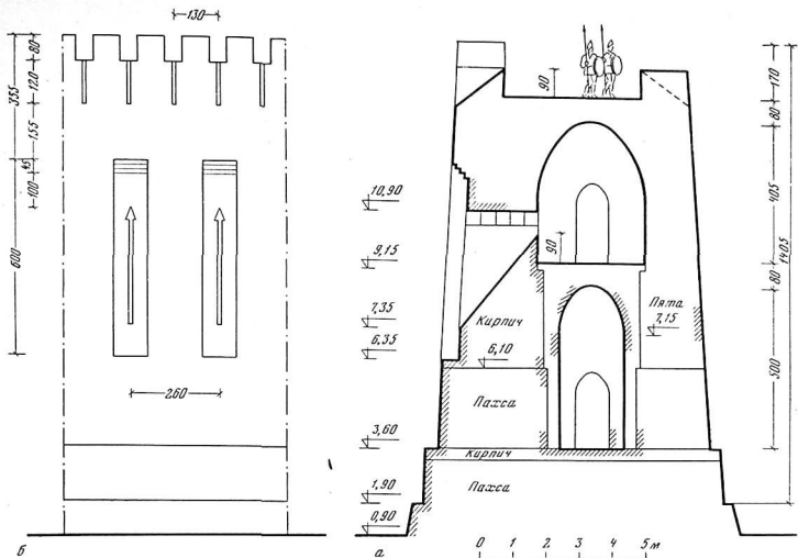
Рис. 32. Крепостная стена периода I. Реконструкция а — поперечный разрез (заштрихованы контуры конструкций, зафиксированные на разных участках стен города); отметками обозначены обмерные данные, остальные размеры по вертикали — реконструированные; б — фрагмент фасада
