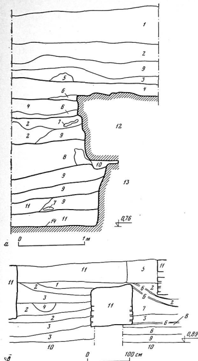
Рис. 5. Разрезы через наслоения к квартале Б
