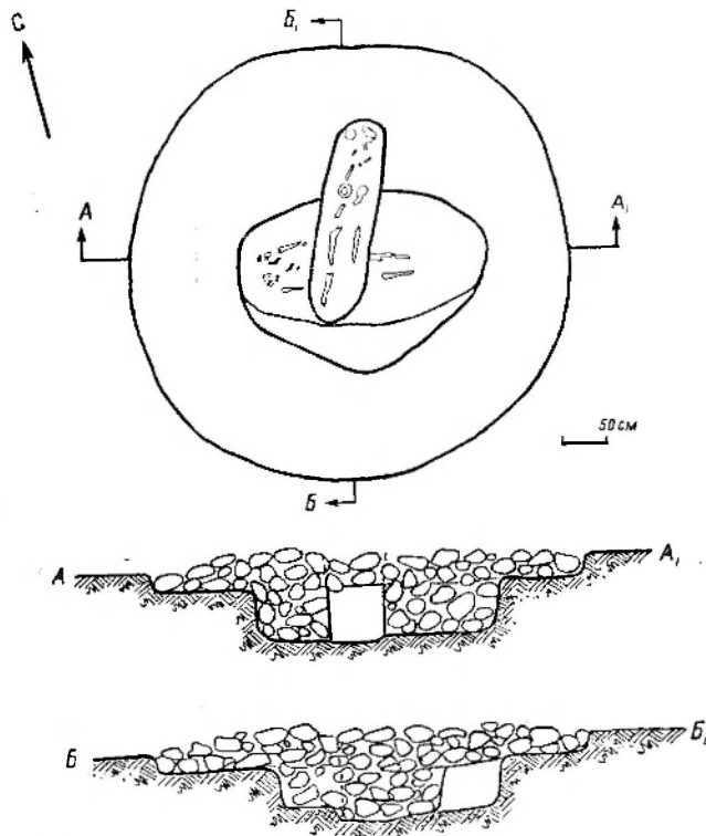
Рис. 6. Ак-тамский могильник. Курган 80, план и разрез. А и Б — линии разрезов.
