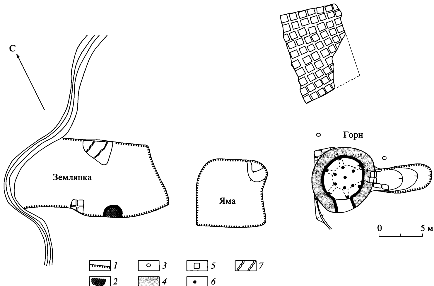
Рис. 6. Гончарная мастерская в пригороде Кампыртепа: 1 – борт котлована, вырубленного в материке; 2 – зольник; 3 – столбовая ямка; 4 – кирпичные стены обжигательной камеры; 5 – сырцовый кирпич; 6 – продухи; 7 – пахса.
