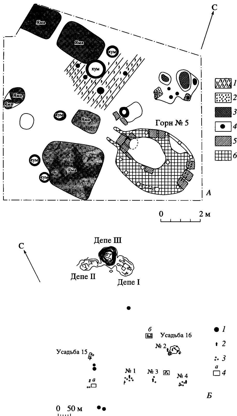
Рис. 3. Нурумское поселение. А – горн № 5 Нурумского поселения: 1 – разрушенная кладка сырцовых кирпичей; 2 – пережженный гипс; 3 – зольники; 4 – столбовая ямка; 5 – сырцовые кирпичи; 6 – прокаленная поверхность пода обжигательной камеры. Б – план центральной части Нурумского поселения: 1 – обжигательный горн; 2 – винодавиля; 3 – стационарно установленные хумы; 4 – отдельные небольшие постройки.
