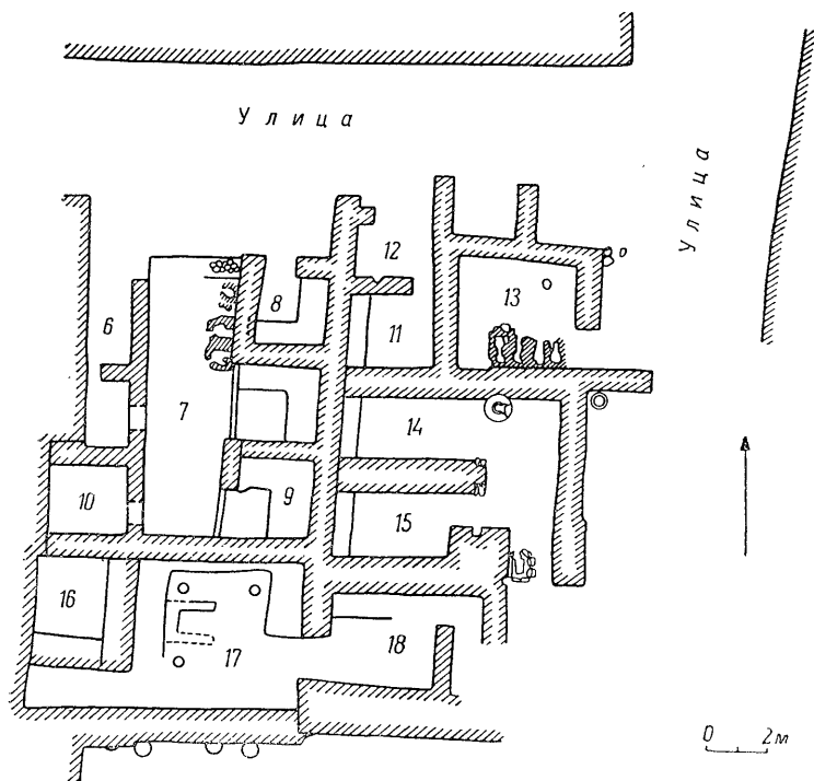
Рис. 49. Пенджикент. План базарчика у перекрестка улиц 1 и 2.
