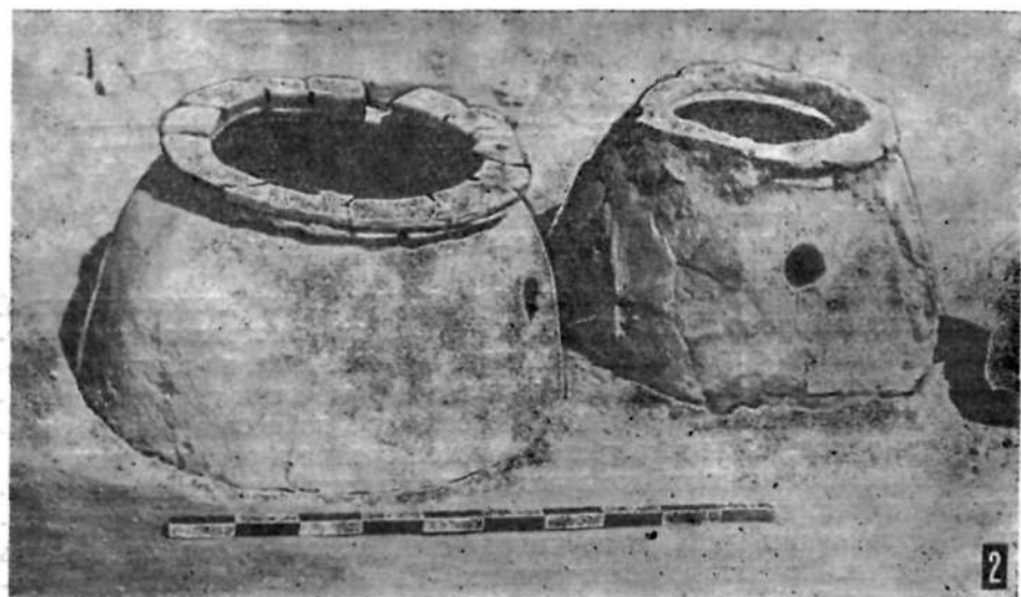
Рис. 27. Танды после снятия суфы: 1 — вид со стороны топки; 2 — вид со стороны дымоходов
